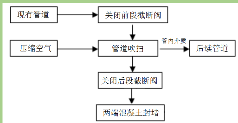
图 2-5 原有管道处理流程图
