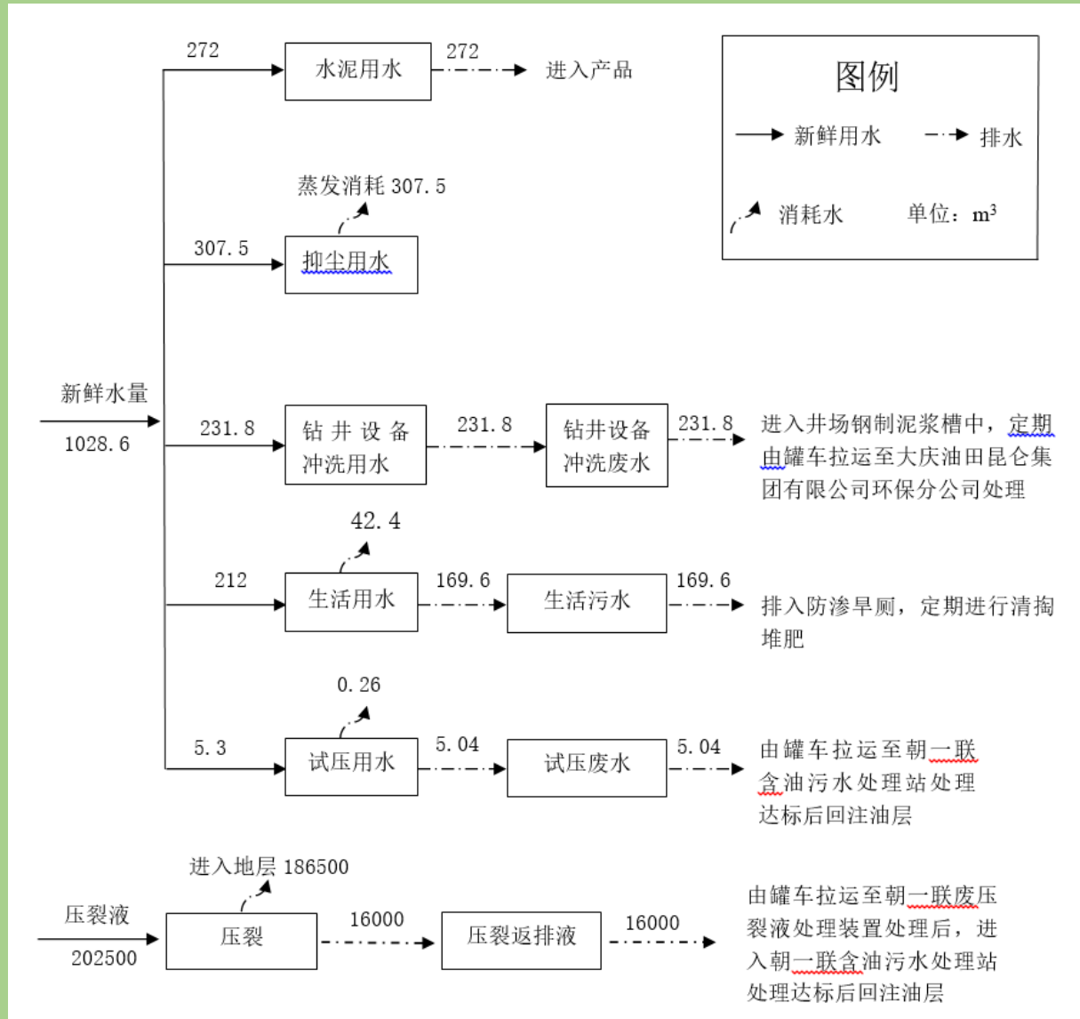
图 3.5-2 施工期水平衡图
