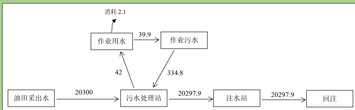
图 3.5-3 运营期水平衡图（单位 \text{m}^3/\text{a} ）
