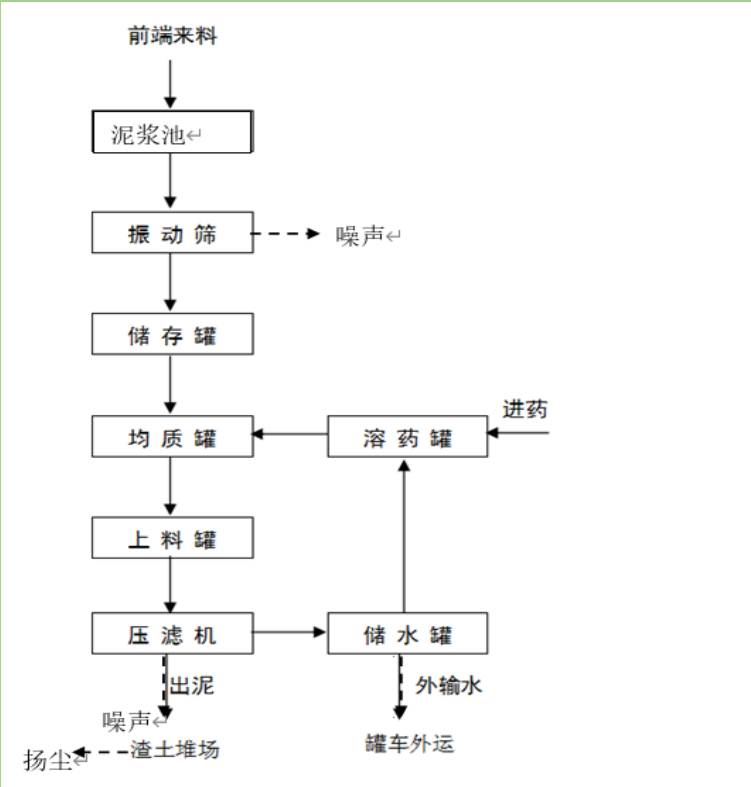
图 3.10-1 大庆油田昆仑集团有限公司环保分公司工艺流程图
