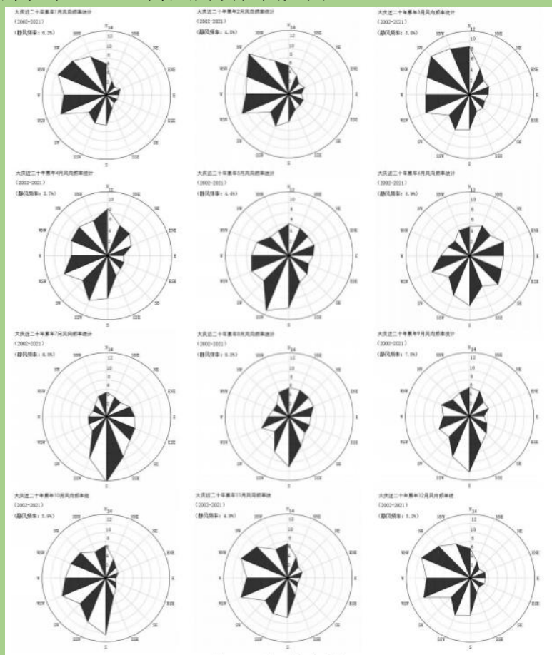
图 5.1-3 月风向玫瑰图（静风频率 5.5%）
