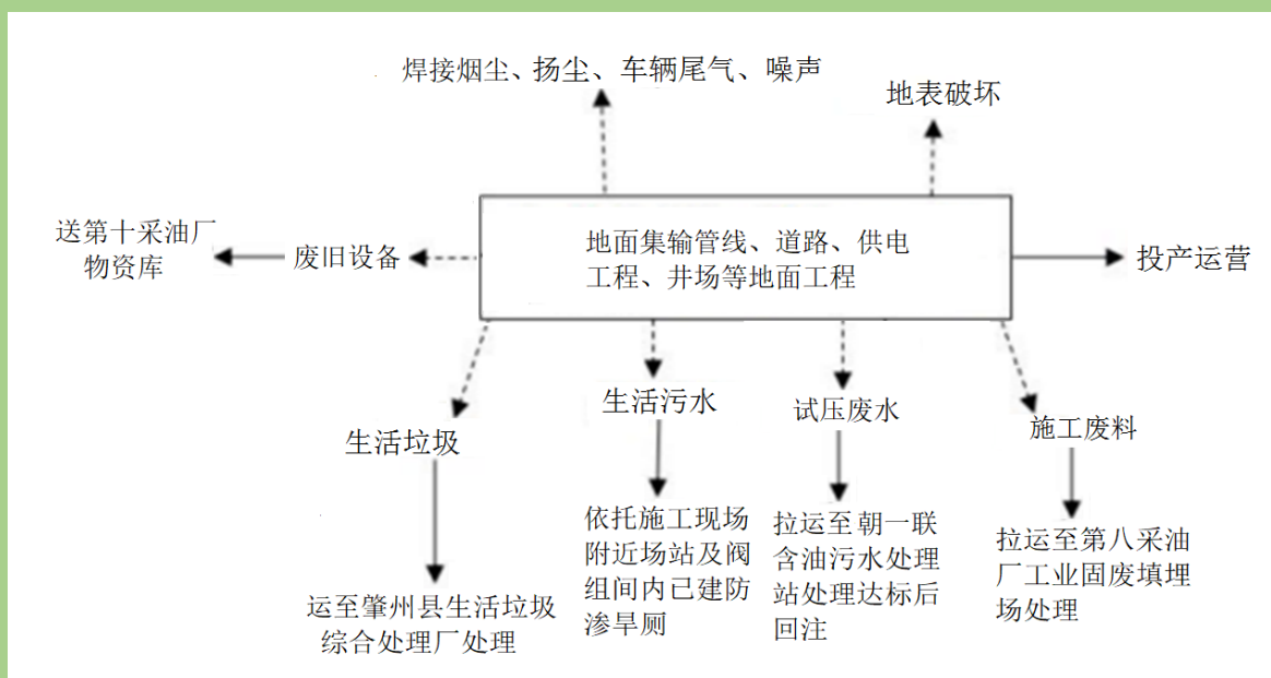
图 3.11-2 本项目地面工程施工期产污环节图
