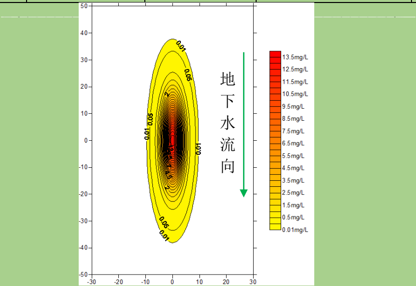
图 5.3-1 集油管道泄漏后 100 天污染物浓度分布图（污染源点：0，0）
