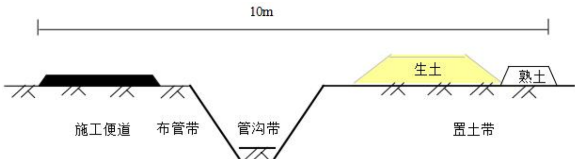
图 3.1-3 管道施工断面布置图
