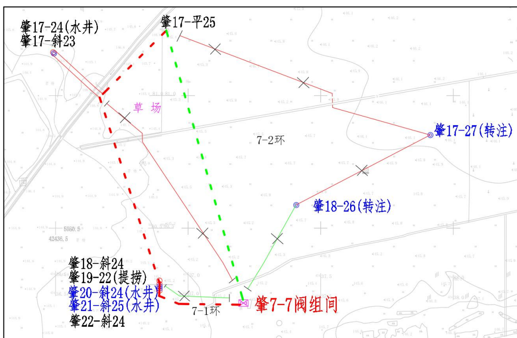
图 3-1-6 肇 1-7 集油阀组间 4 环管道优化后管道走向示意图
