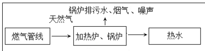
图 2-3 运营期加热炉、锅炉产污节点图
