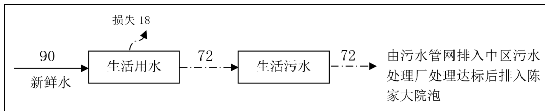
图 2-5 项目厂区水平衡分析图 (单位: m 3 /a)
