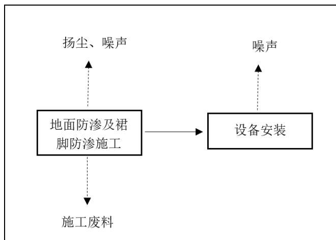
图 2-6 本项目施工期工艺流程图及产污节点
