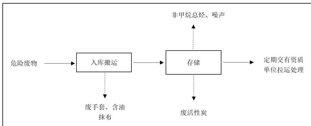
运营期工艺流程及产污节点图
