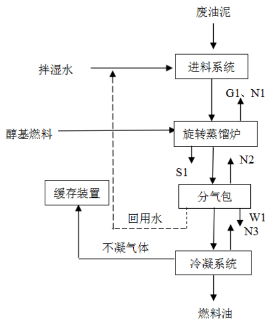
图 3.10-5 大庆博昕晶化科技有限公司工艺流程图
