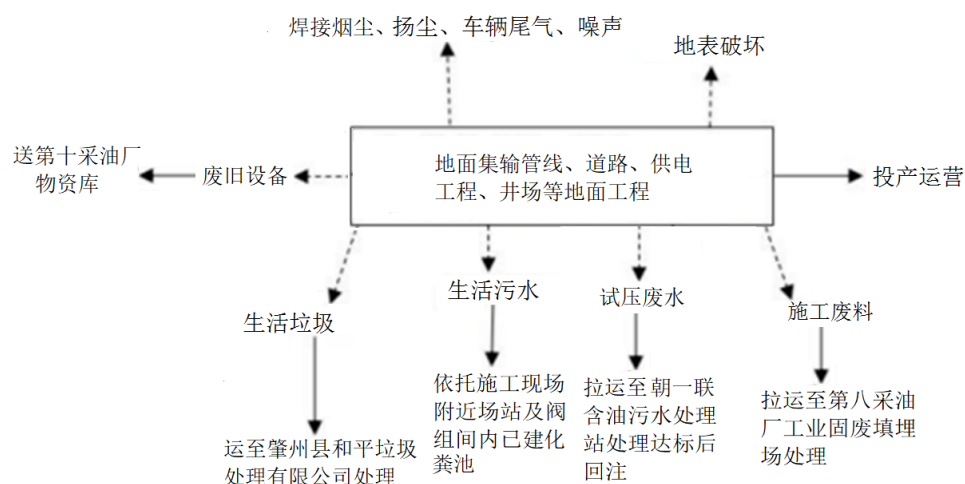
图 3.11-4 本项目地面工程施工期产污环节图
