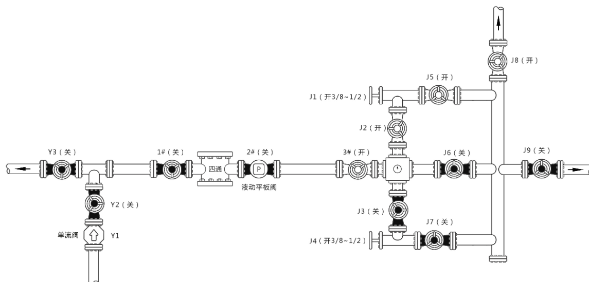
图 3.5-4 二开、三开节流管汇及压井管汇示意图
