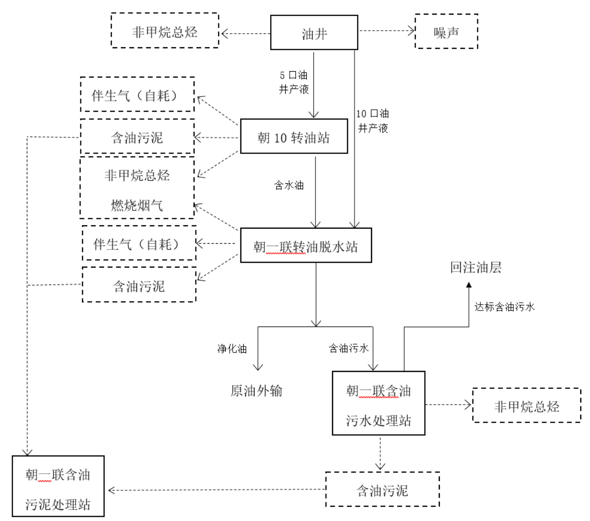
图 3.11-5 运营期正常工况工艺流程及产污示意图
