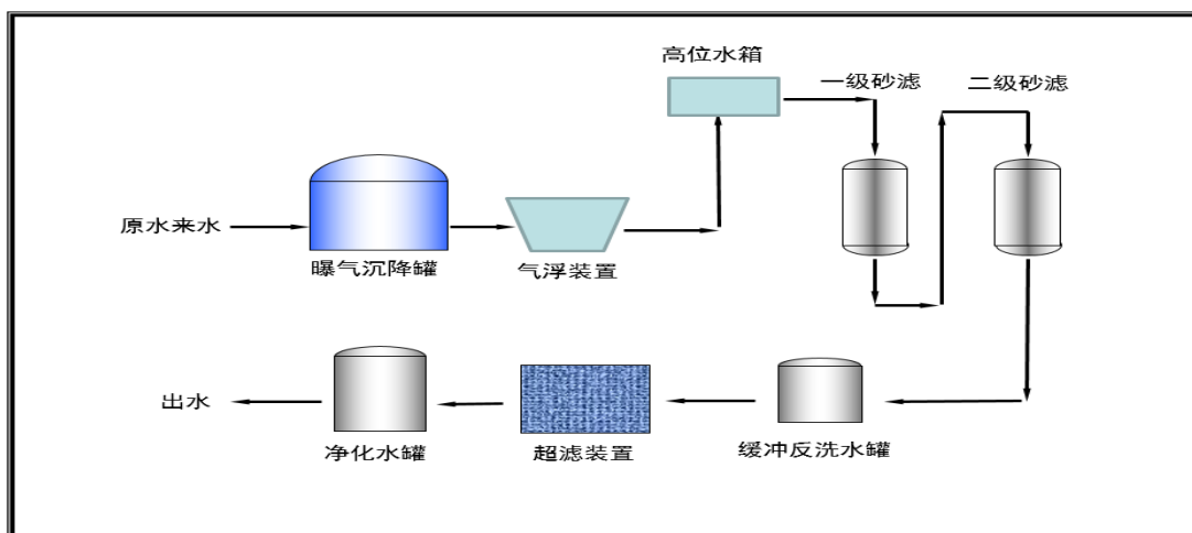
图 3.10-3 龙一联合含油污水处理站工艺流程
