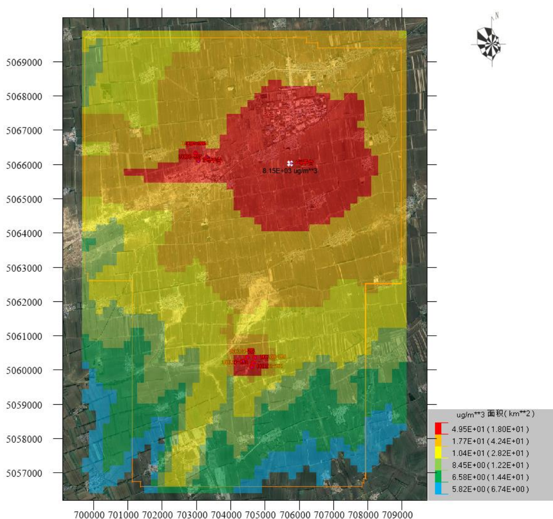
图 5.1-21 非正常工况废气污染物预测结果图
