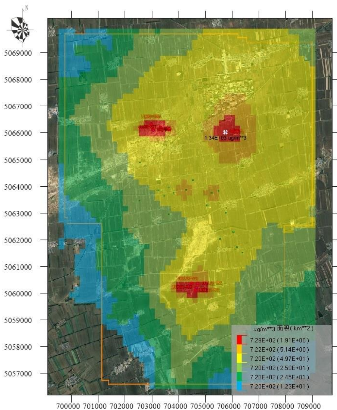
图 5.1-20 新增污染源+在建污染源叠加背景值后 NMHC 小时值浓度分布图
