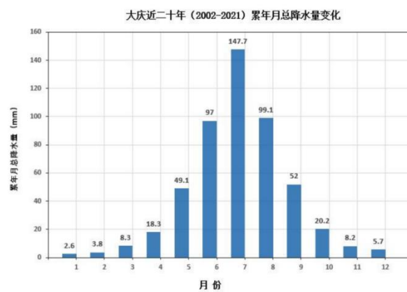
图 5.1-7 月平均降水量（单位：毫米）
