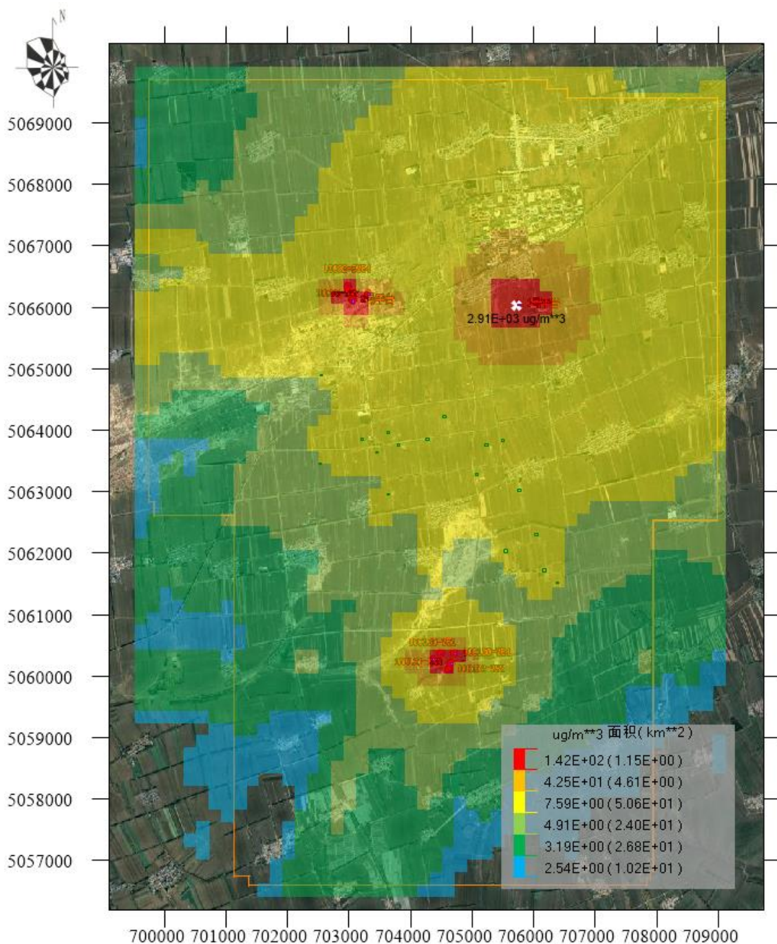
图 5.1-19 新增污染源及其他在建污染源 NMHC 小时值贡献浓度分布图
