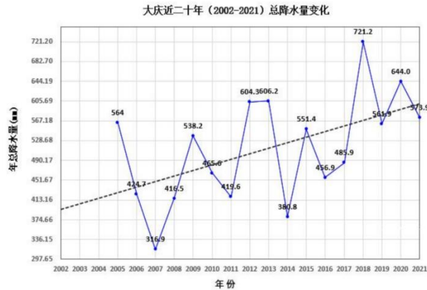
图 5.1-8 （2002-2021）年总降水量（单位：毫米，虚线为趋势线）
