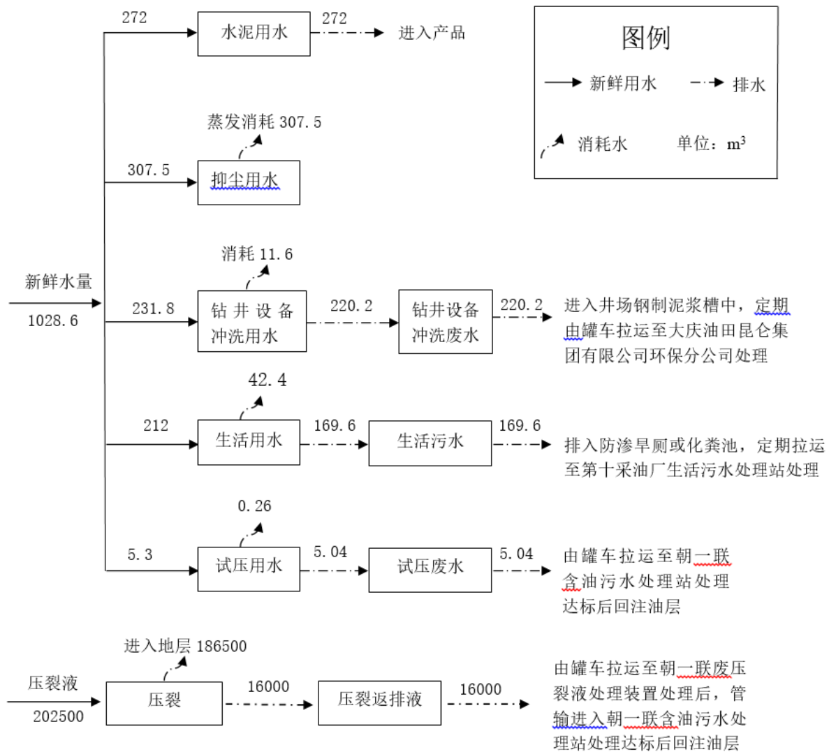
图 3.5-6 施工期水平衡图
