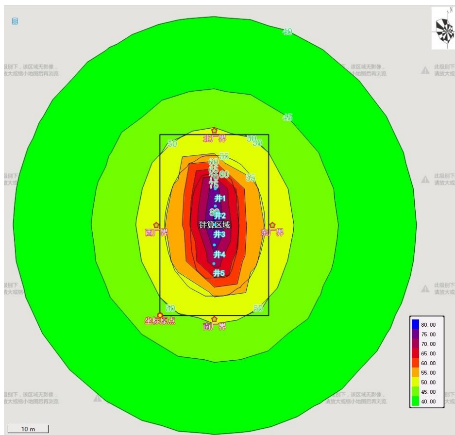
图 5.4-3 1 号平台井场厂界噪声预测结果图
