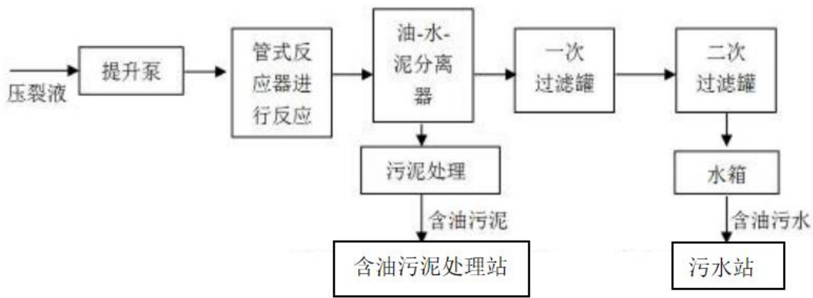
图 3.10-7 龙一联压裂返排液处理站工艺流程图
