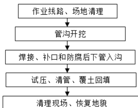
图 3.7-2 管道施工建设过程
