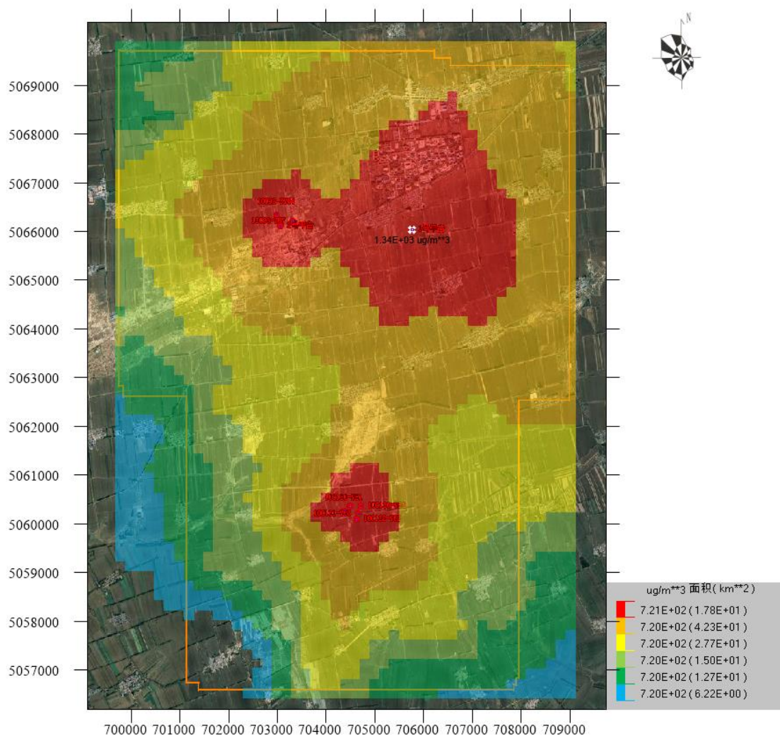
图 5.1-18 叠加背景值后 NMHC 小时浓度分布图
