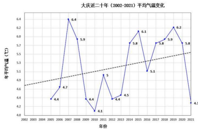
图 5.1-6 （2002-2021）年平均气温（单位：℃，虚线为趋势线）
