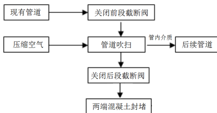
图 3.11-2 原有管道处理流程图
