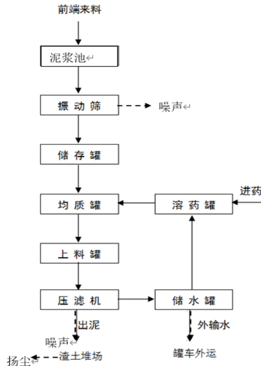
图 3.10-6 大庆钻探六号废弃钻井液处理站（采油九厂）工艺流程图
