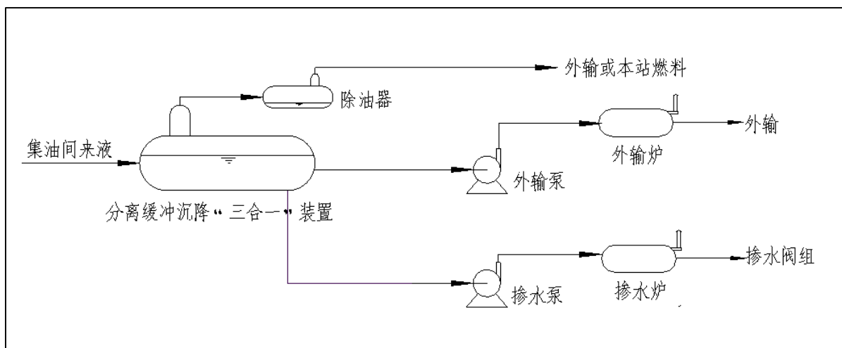
图 3.10-1 塔一转油站工艺流程图
