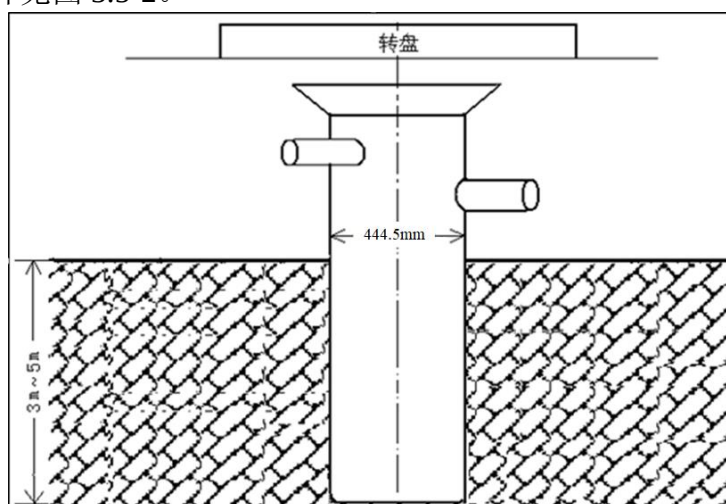
图 3.5-2 一开井口装置设计示意图
