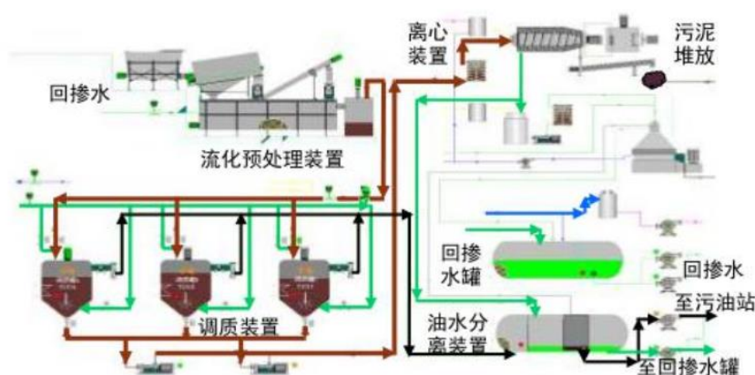
图 3.10-4 第九采油厂含油污泥处理站工艺流程图
