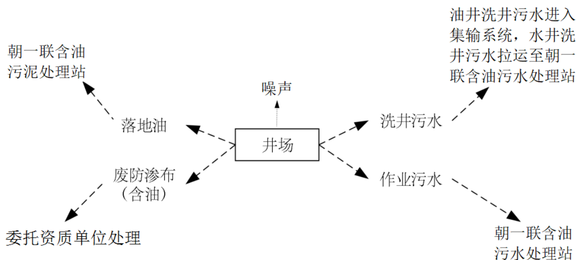
图 3.11-6 运营期非正常工况工艺流程及产污示意图
