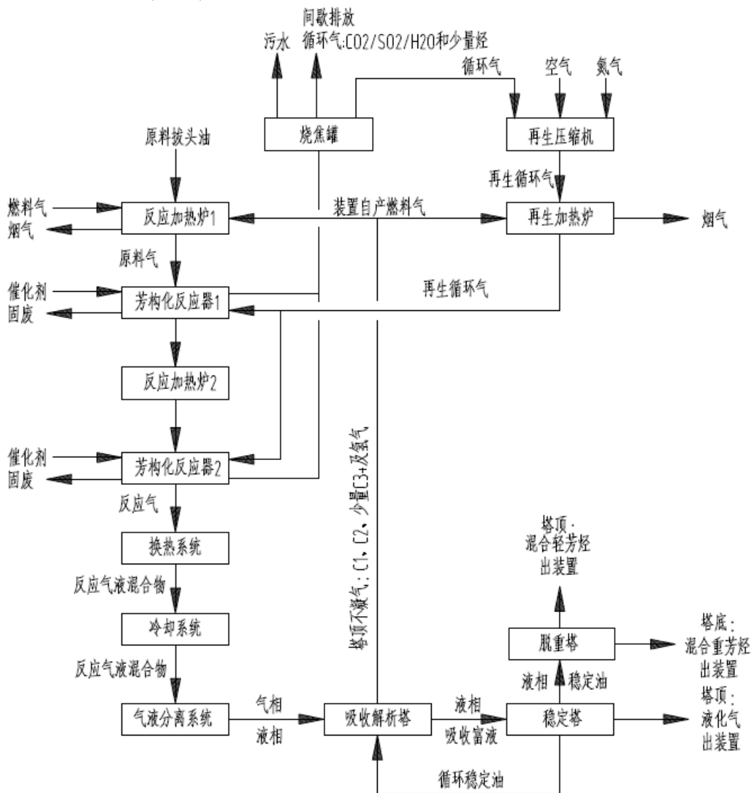
图 3.1-3 15万吨/年轻烃芳构化工艺流程及产污节点图
