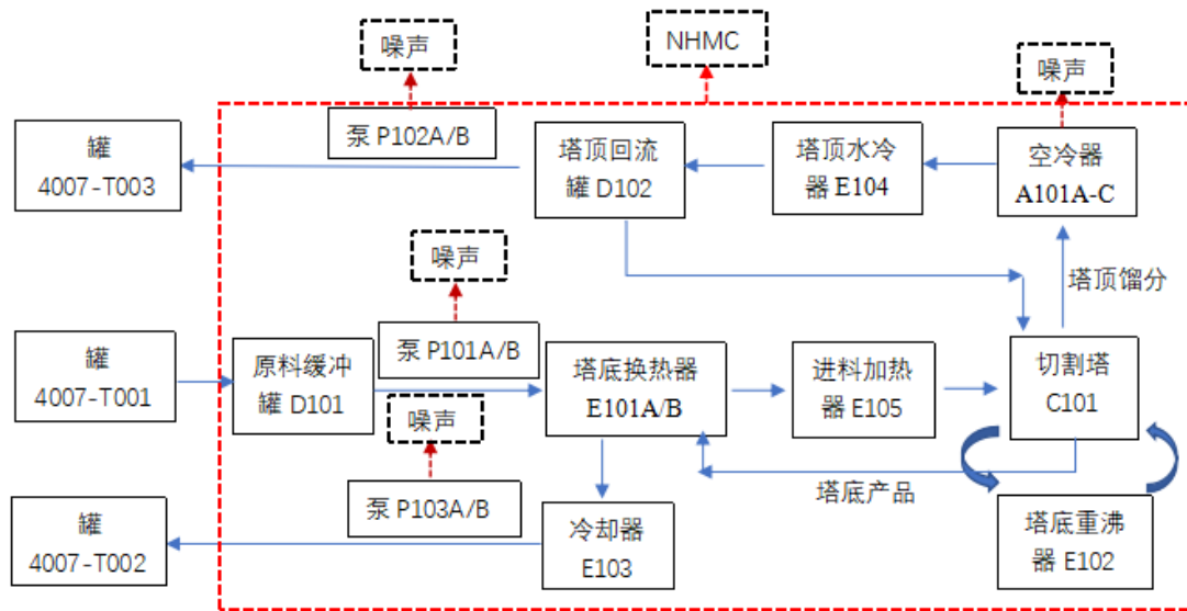
图3.2-4 工艺流程产污环节图
