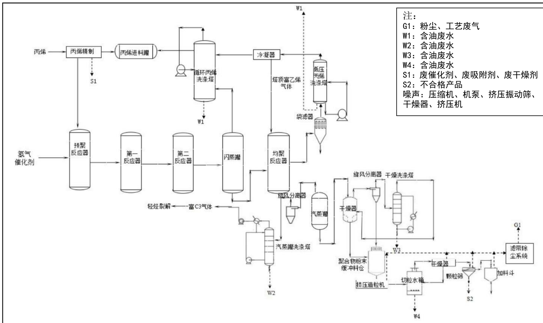
图 3.1-15 聚丙烯装置生产工艺流程及排污节点图
