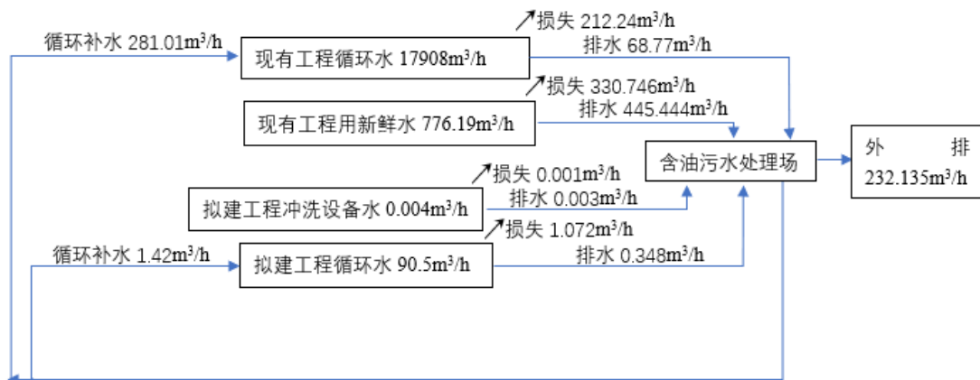
图 3.2-3 工程水平衡图
