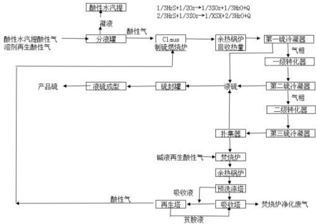
图 3.1-21 硫磺回收装置工艺流程图
