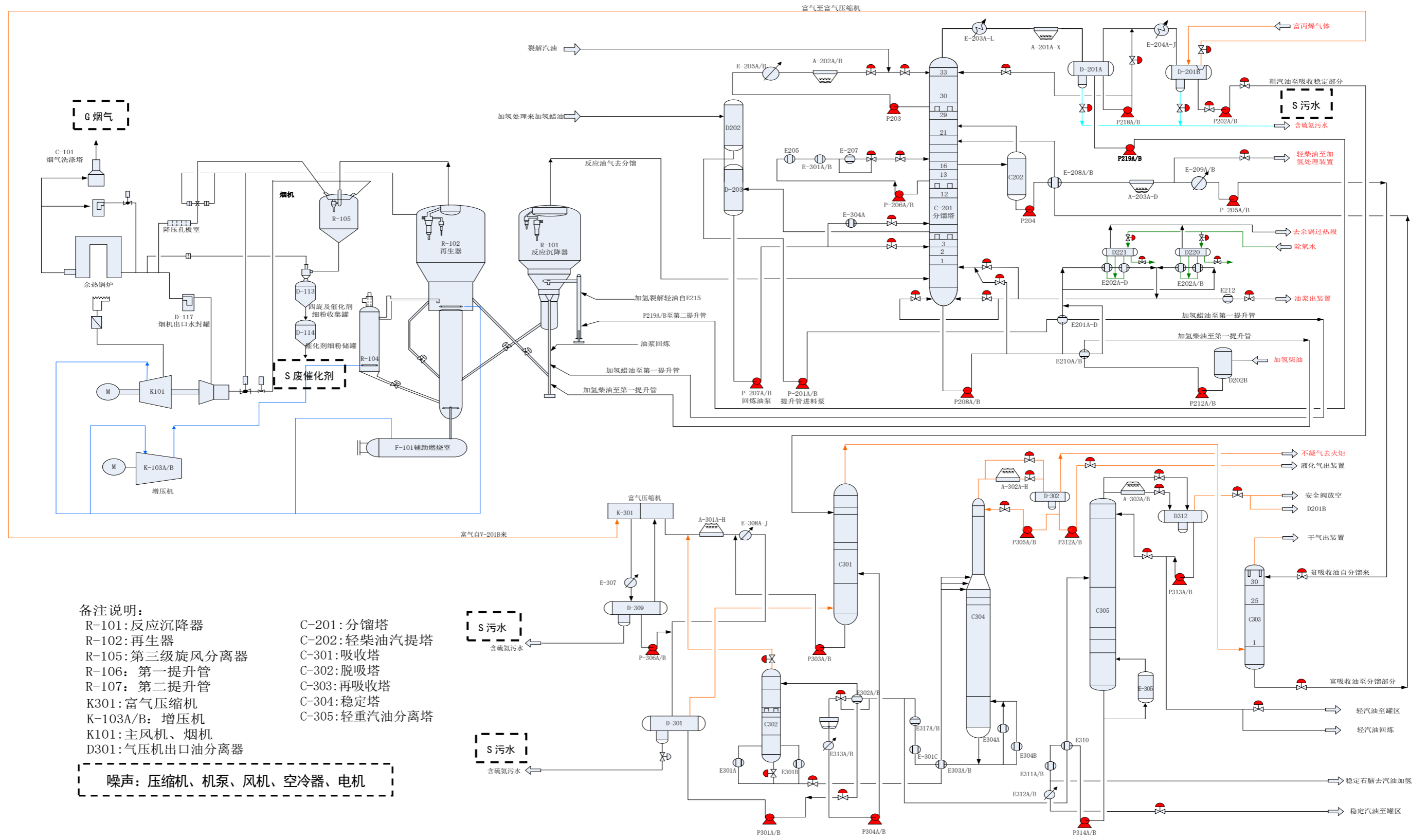
图 3.1-2 (2) 230 万吨/年催化热裂解 (DCC 装置) 工艺流程及产污节点图
