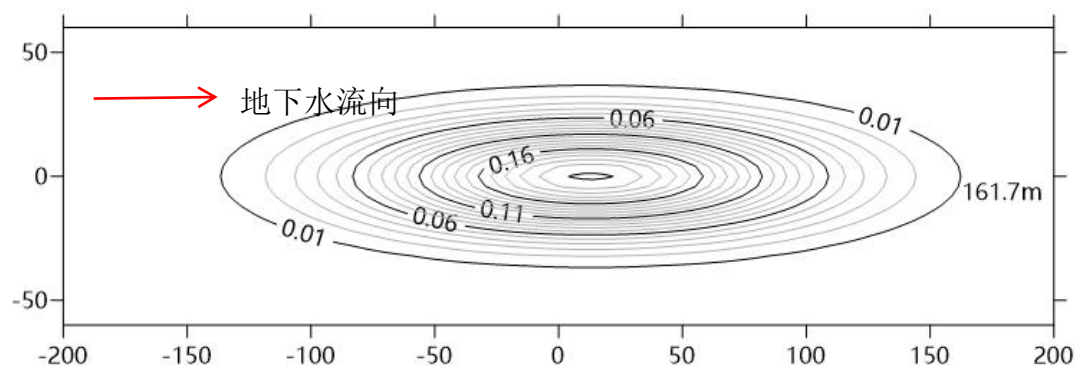
图 5.4-6 非正常工况切割塔泄漏 3650d 石油类影响分布图
