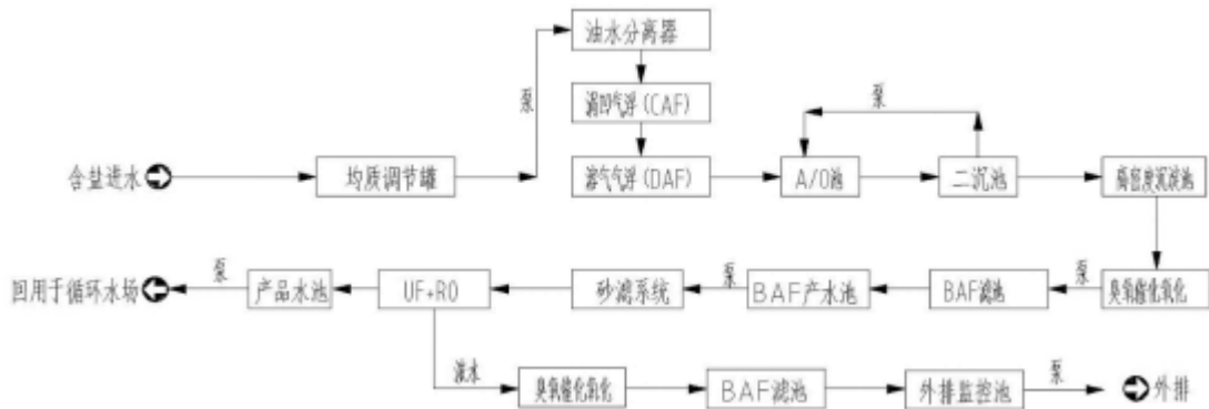
图 3.1-25 污水处理场含盐系列处理工艺流程图
