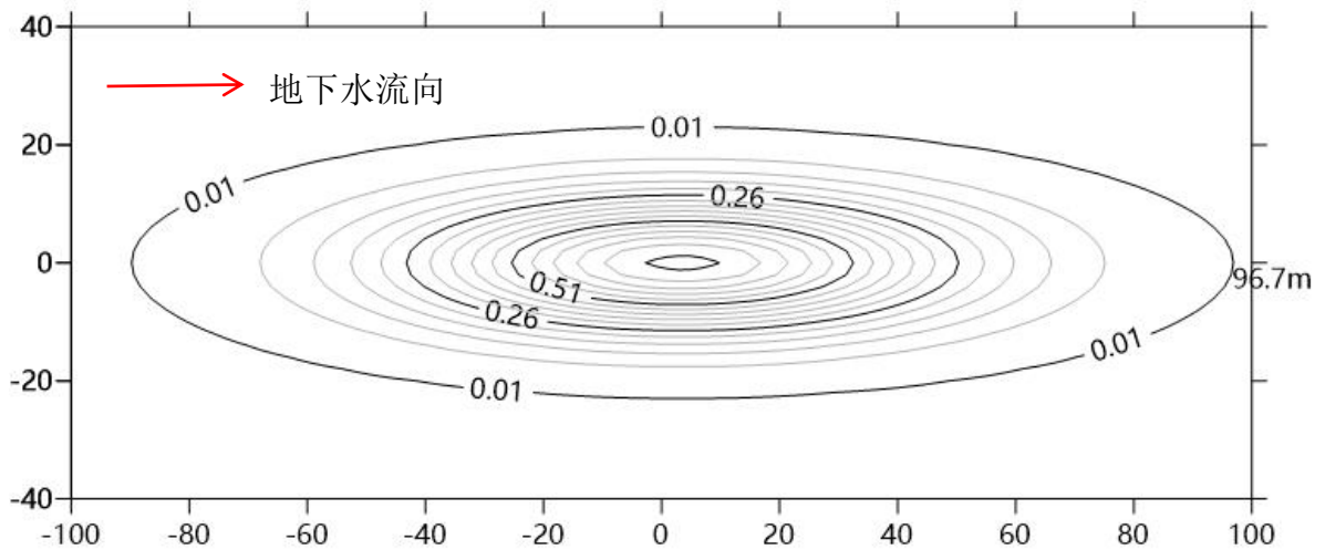
图 5.4-3 非正常工况切割塔泄漏 1000d 石油类超标分布图
