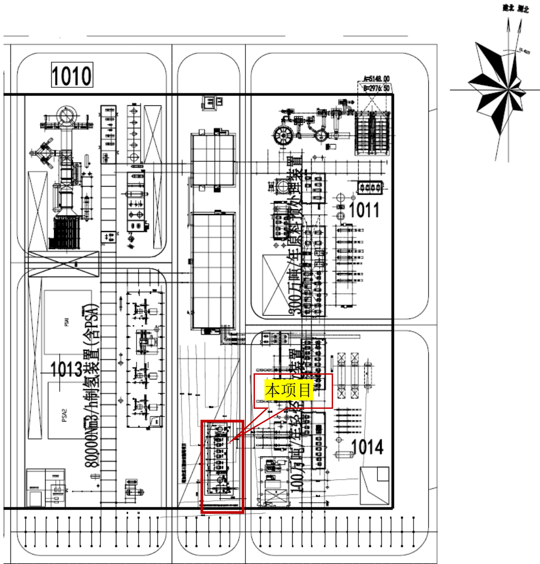
图 3.2-1 项目平面布置图
