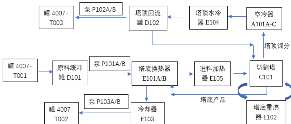
图 3.2-2 项目工艺流程图
