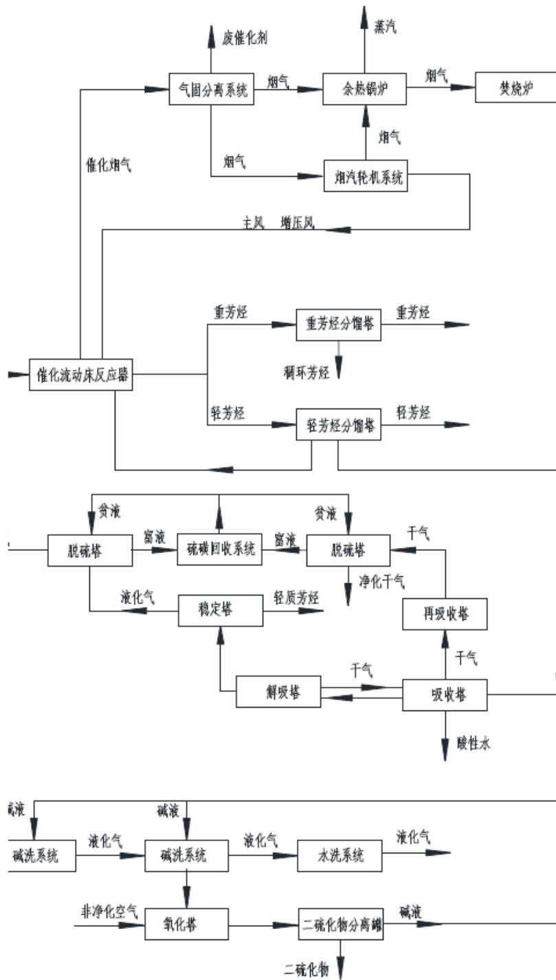
图 3.1-2 (1) 230 万吨/年催化热裂解 (DCC 装置) 工艺流程及产污节点图
