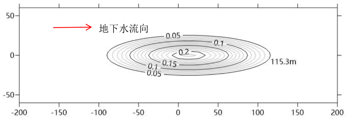
图 5.4-5 非正常工况切割塔泄漏 3650d 石油类超标分布图
