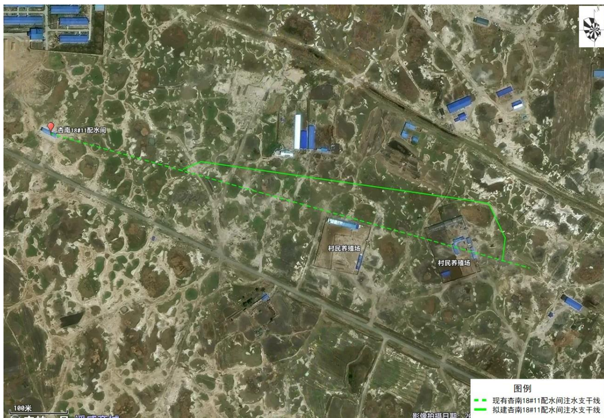
图 3.4-2 拟建注水支干线管道走向图
