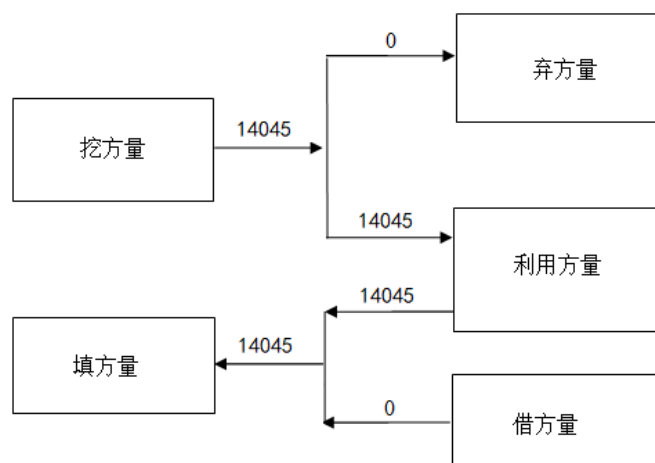
图 3.5-1 土石方平衡图 (单位: \text{m}^3 )
