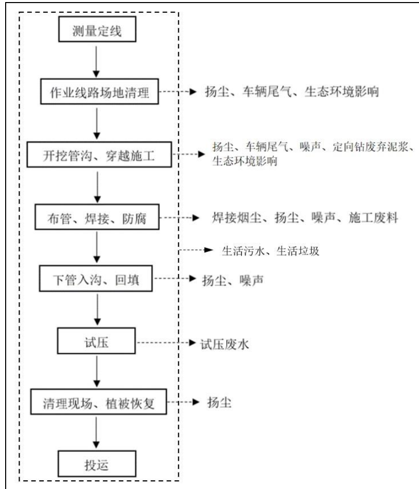
图 3.10-2 管线施工工艺流程及产污节点图
