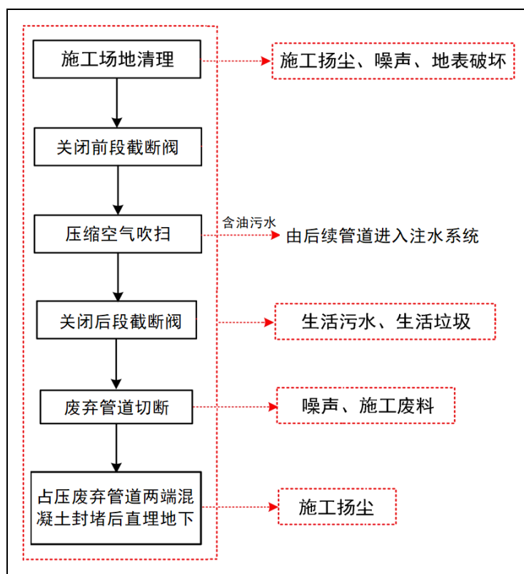
图 3.10-1 原有管道处理工艺及产污节点图
