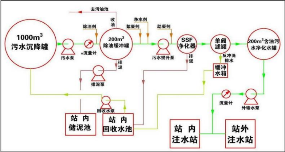
图 3.9-1 杏 V-1 联合油污水处理站工艺流程
