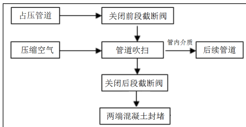
图 3.6-1 原有管道处理流程图
