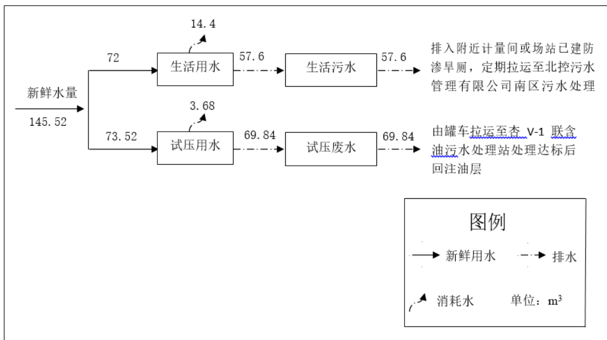
图 3.4-5 施工期水平衡图
