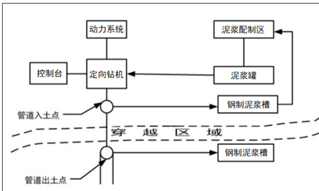
图 3.6-6 定向钻穿越施工平面布置图
