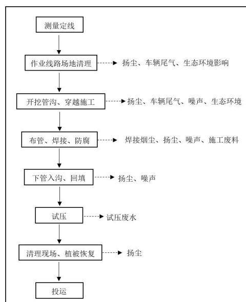
图 3.12-2 管线施工过程示意图
