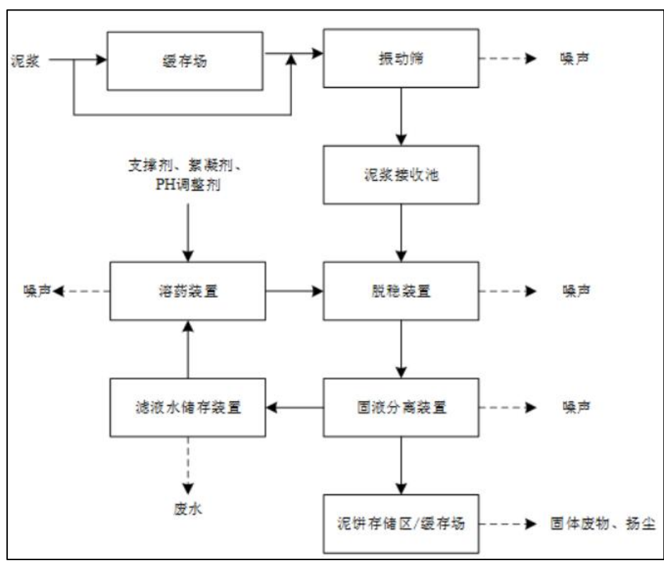
图 3.11-7 大庆市四厂废弃钻井液无害化处理站工艺流程图
