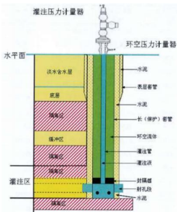
图 5.3-13 注水井井身结构示意图
