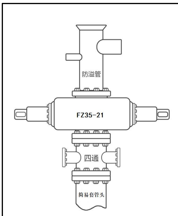
图 3.6-3 二开井口装置示意图
