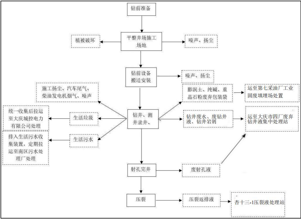
图 3.12-1 本项目钻井及井下作业工艺流程及产污环节图
