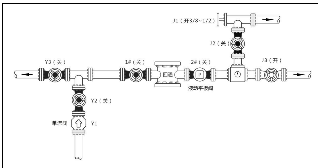
图 3.6-4 二开节流管汇示意图
