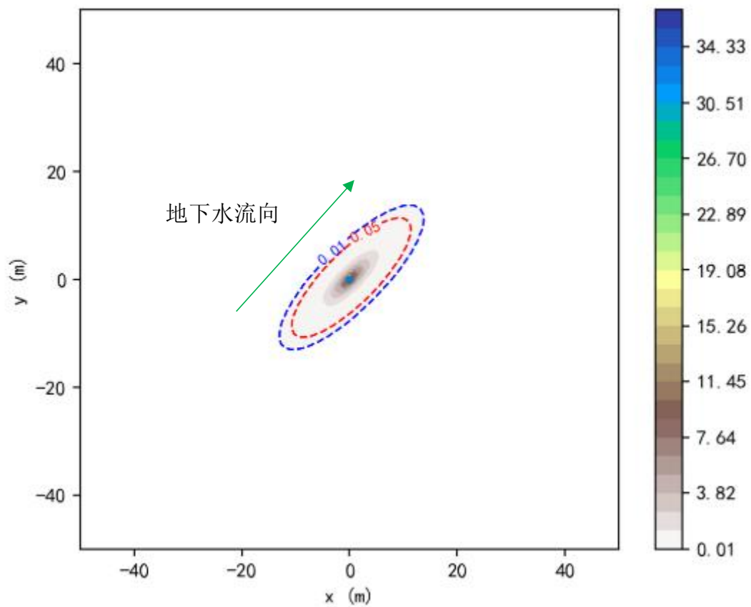
图 5.3-14 注水井套管泄漏 100 天石油类污染扩散平面图（污染源点：0，0）
