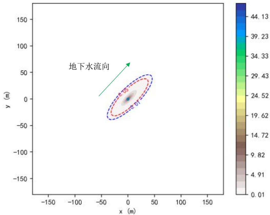
图 5.3-15 注水井套管泄漏 1000 天石油类污染扩散平面图（污染源点：0，0）
