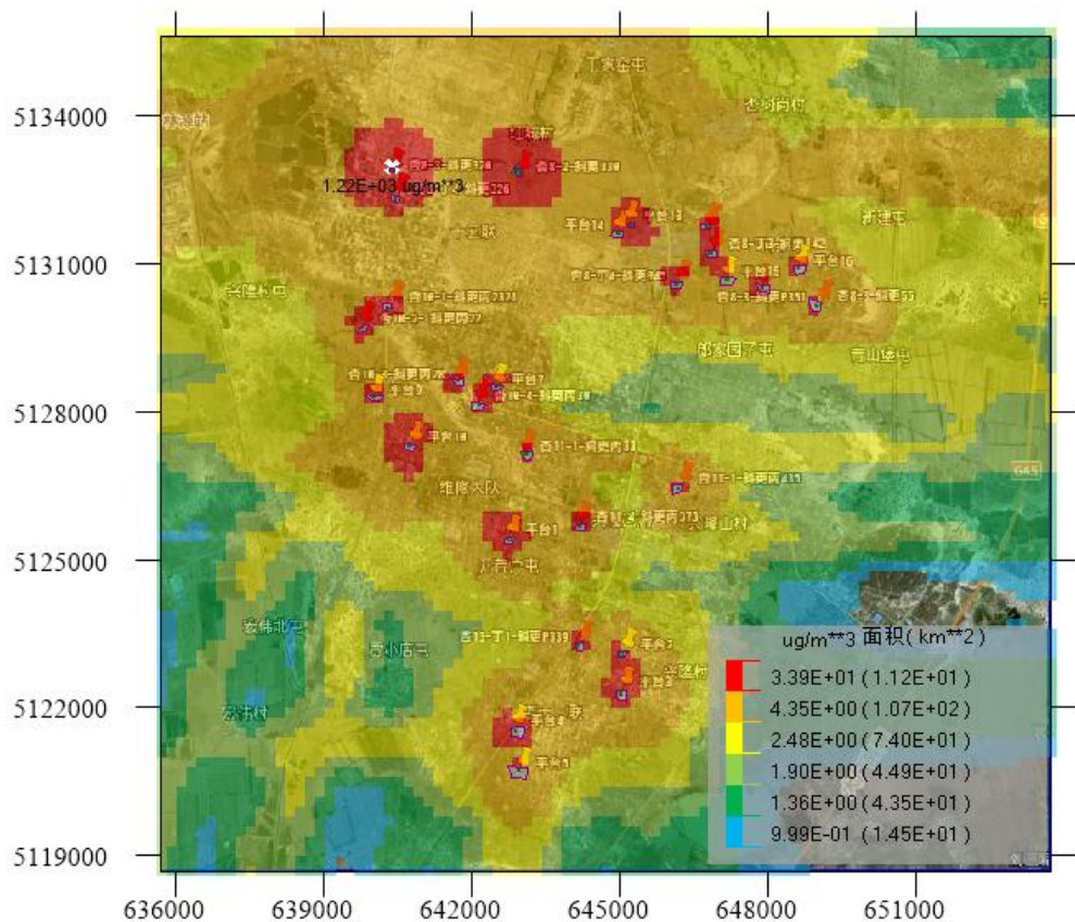
图 5.1-19 非正常工况废气污染物预测结果图
