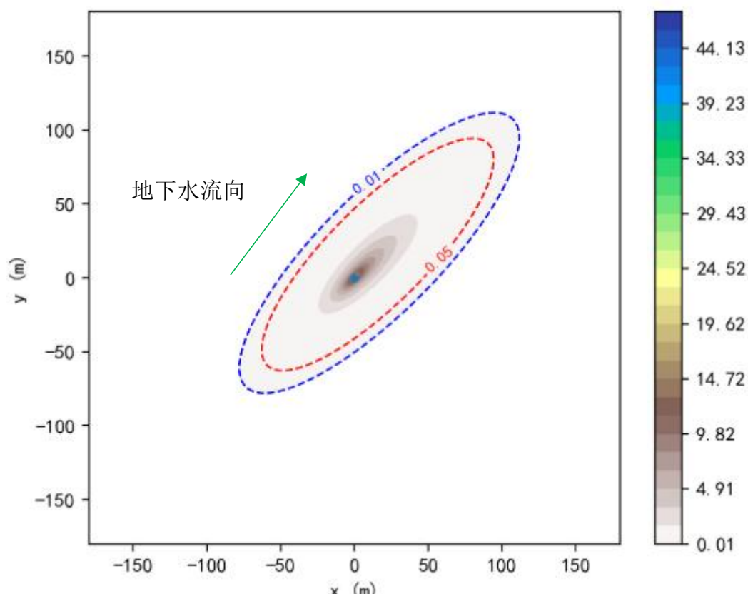
图 5.3-16 注水井套管泄漏 5000 天石油类污染扩散平面图（污染源点：0，0）
