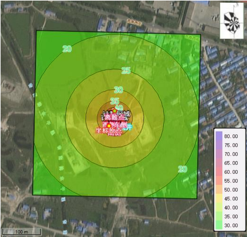
图 5.4-3 杏 11-4-斜更丙 373 井场平台井场噪声预测图
