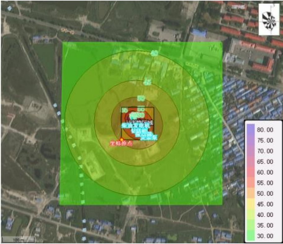
图 5.4-2 钻井施工期井场噪声保护目标处预测图
