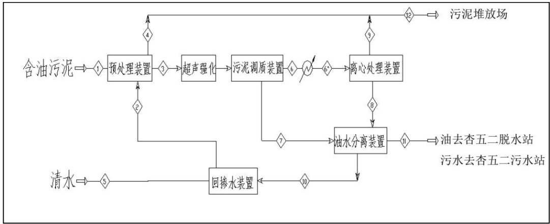
图3.9-5 杏 V- II 含油污泥处理站工艺流程图
