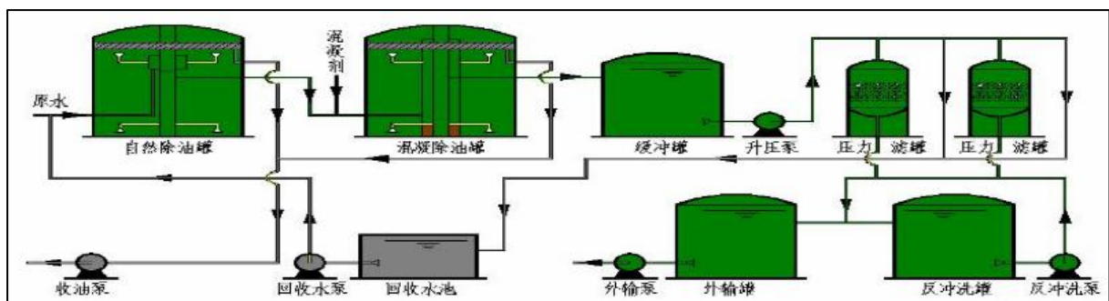
图3.9-3 含油污水处理站工艺流程
