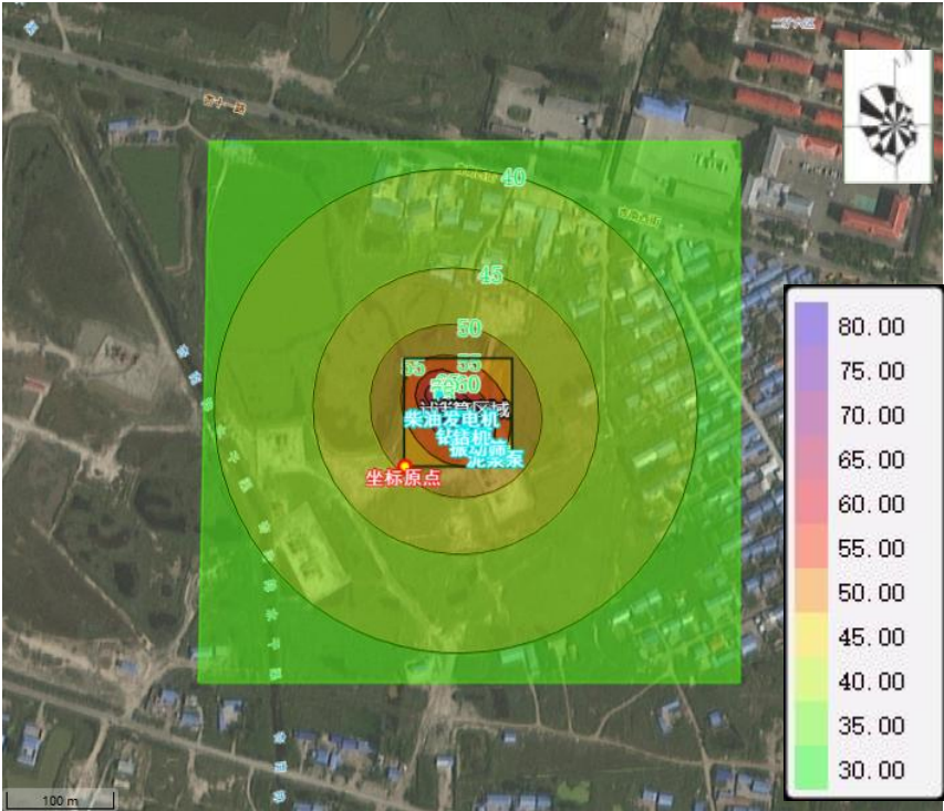
图 5.4-1 钻井工程噪声贡献值预测图
