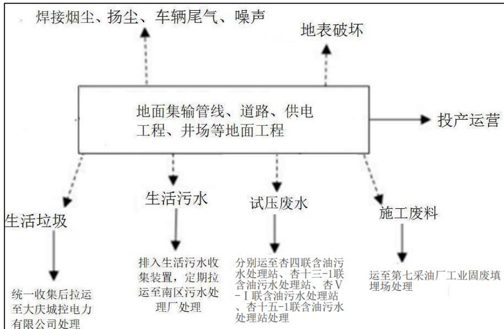
图 3.12-4 本项目地面工程施工期产污环节图
