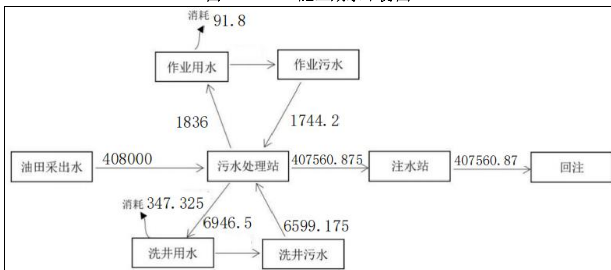
图 3.6-11 运营期水平衡图 (单位 \text{m}^3/\text{a} )
