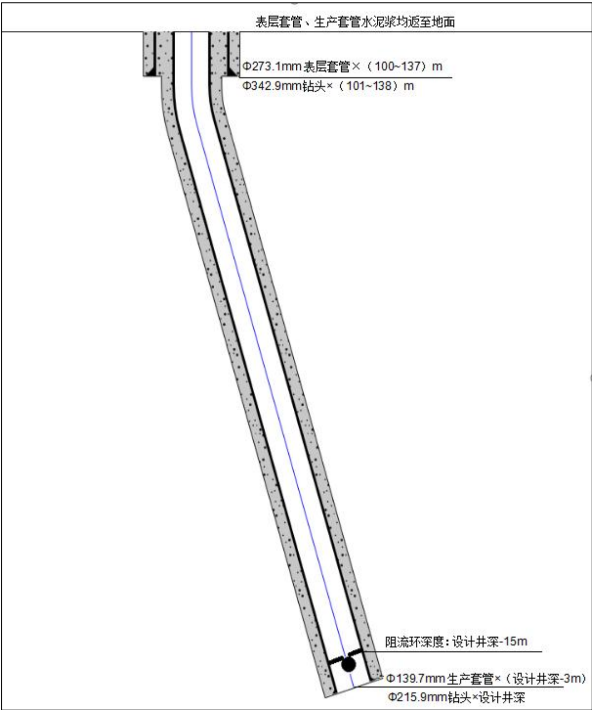
图 3.6-1 井身结构示意图
