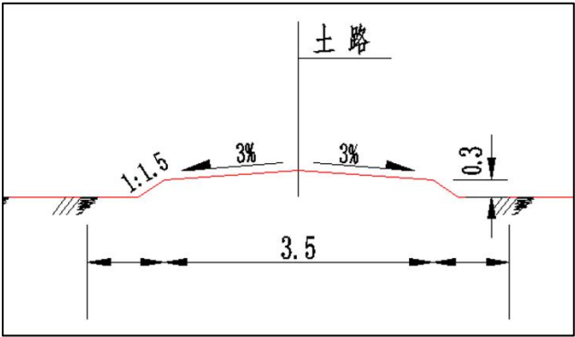
图3.8-6 通井路横断面图
