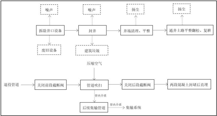
图 3.12-6 退役期工艺流程及主要产污节点图
