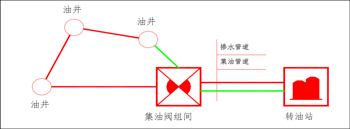
图 3.6-5 单管环状集油工艺流程图
