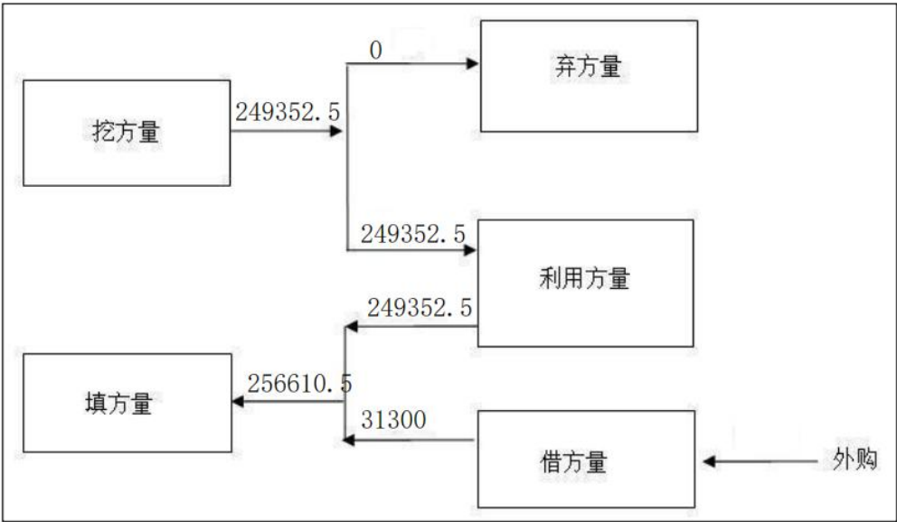
图 3.7-1 土石方平衡图（单位：m³）
