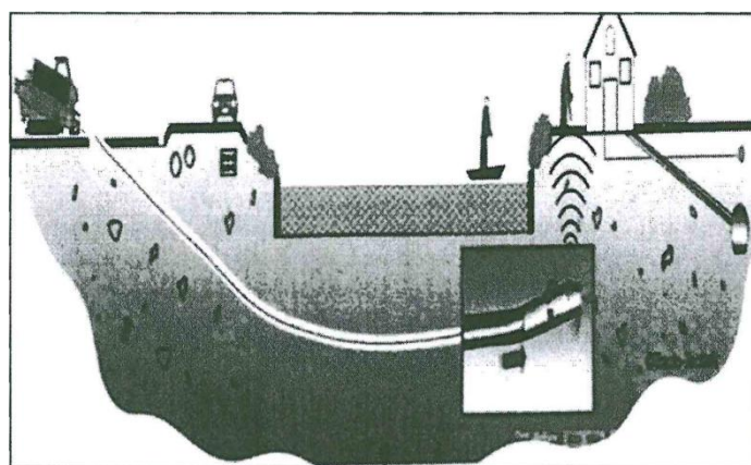
图 3.8-4 定向钻施工示意图
