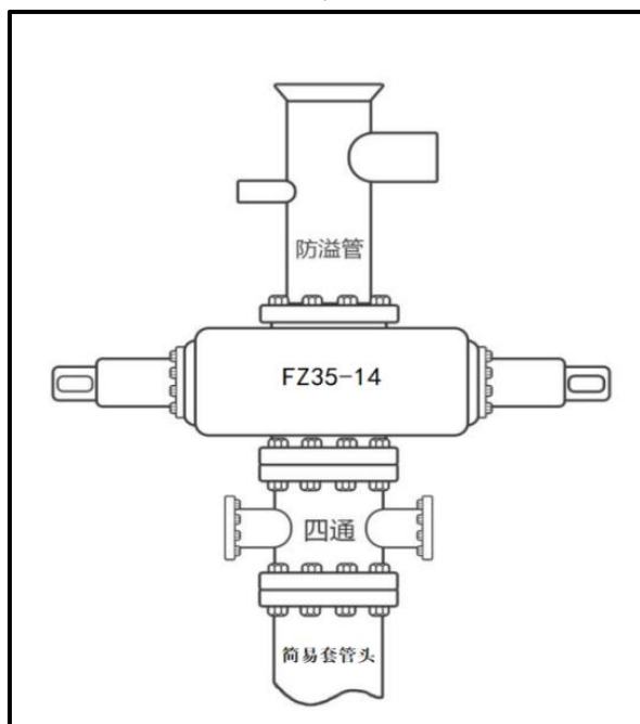
图 3.6-2 二开井口装置设计示意图
