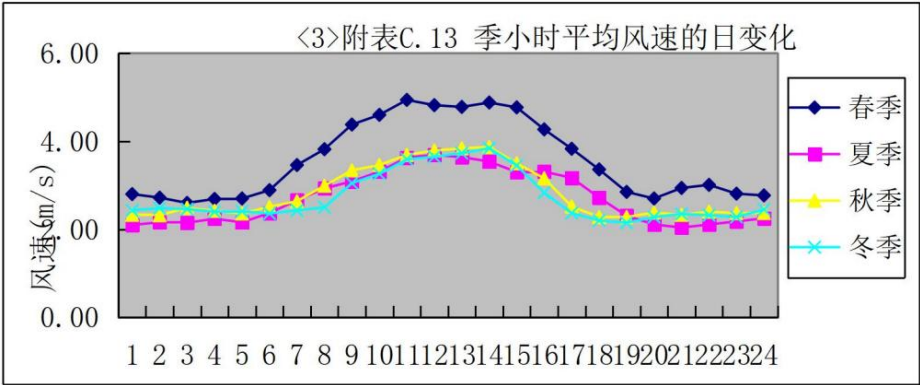
图 5.1-10 年评价区域各季小时平均风速日变化
