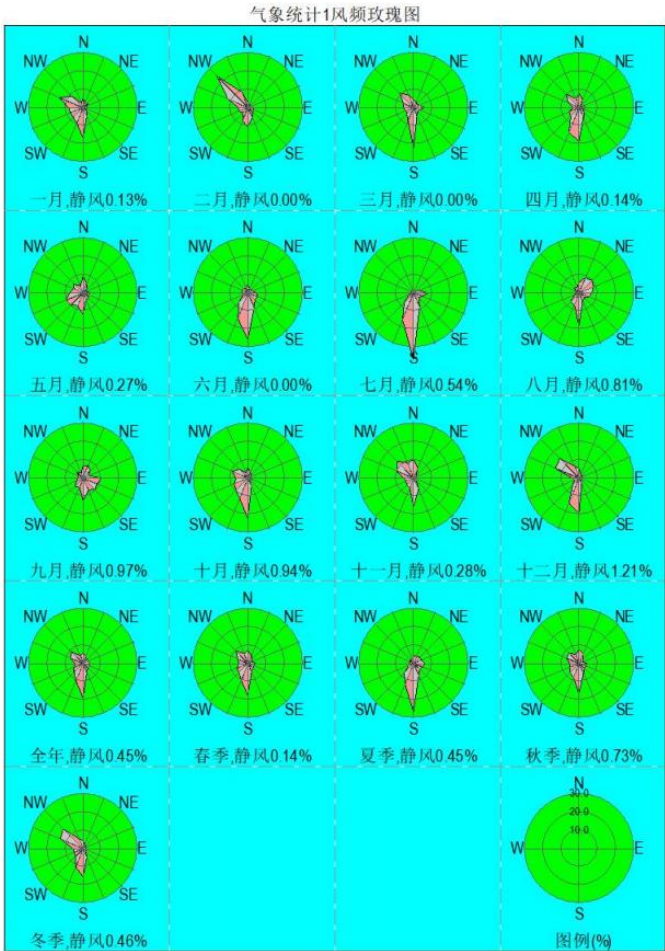
图 5.1-11 2024 年评价区域各月、季及年均风频玫瑰图
