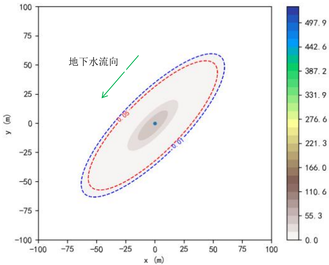
图 5.3-3 集油管道泄漏后 100 天污染物浓度分布图（污染源点：0，0）
