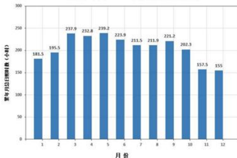
图 5.1-6 月日照时数 (单位: 小时)
