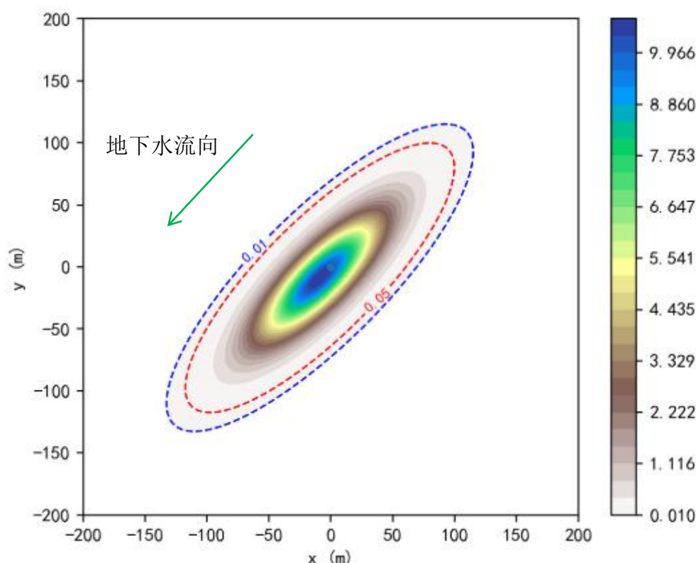
图 5.3-5 集油管道泄漏后 5000 天污染物浓度分布图（污染源点：0，0）
