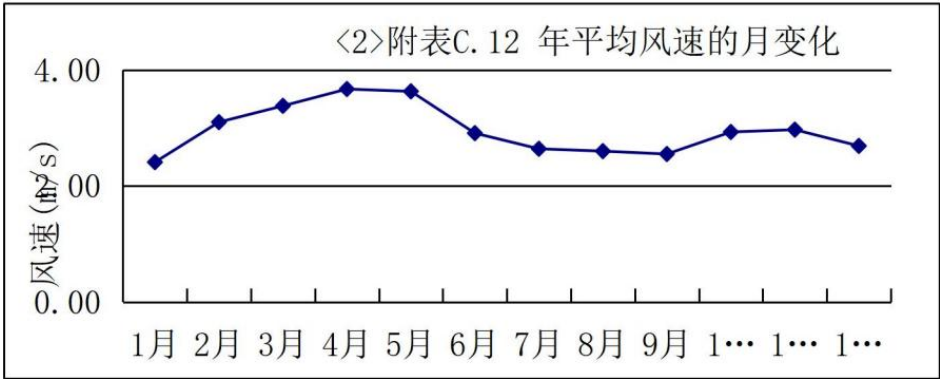
图 5.1-9 2024 年评价区域月平均风速变化图
