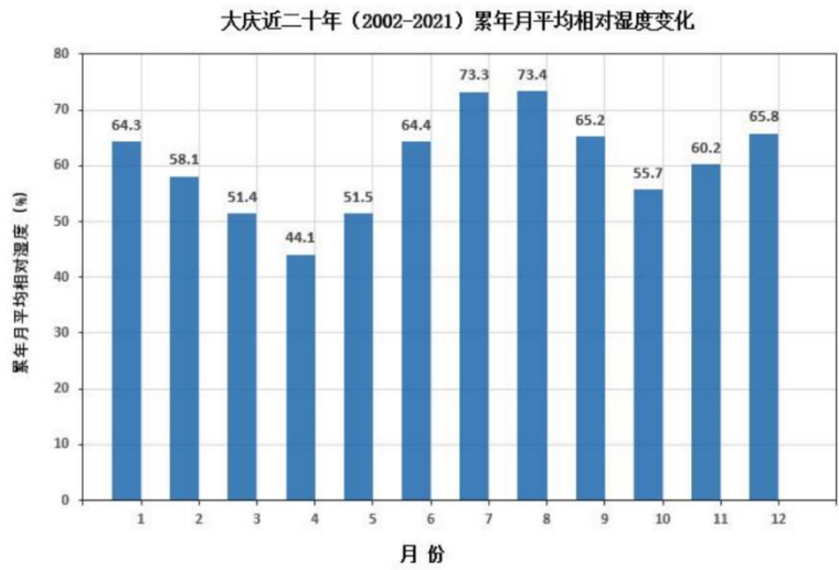
图 5.1-7 月平均相对湿度（纵轴为百分比）
