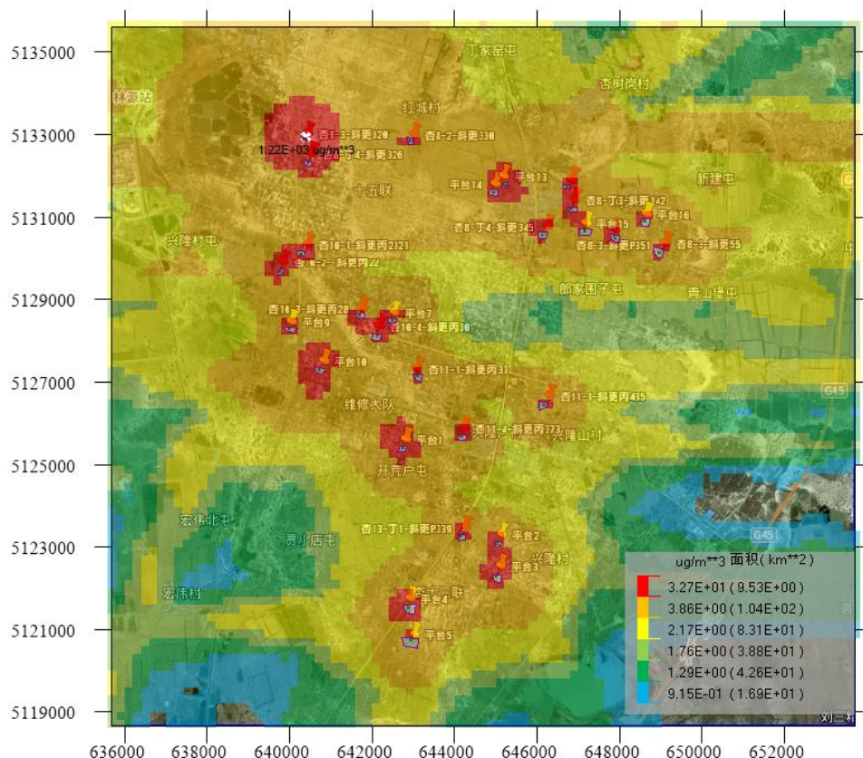
图 5.1-17 NMHC 小时值贡献浓度分布图
