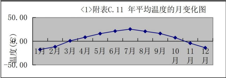
图 5.1-8 2024 年评价区域月平均温度变化图
