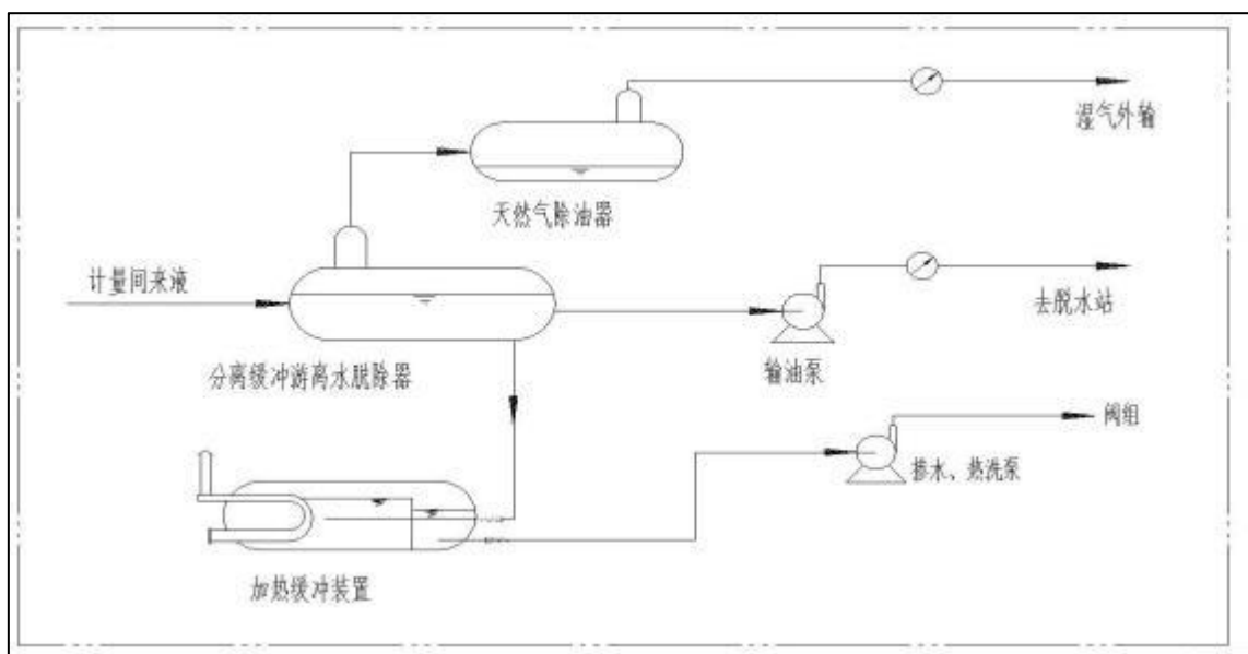
图 3.11-1 转油站工艺流程图
