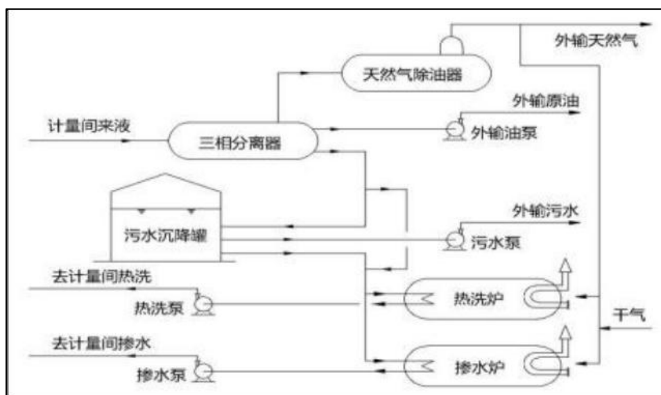
图 3.11-2 转油放水站工艺流程图
