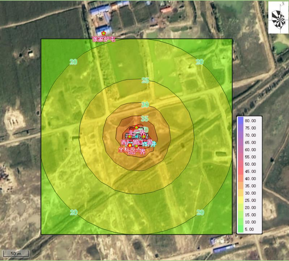
图 5.4-1 运营井场噪声预测图
