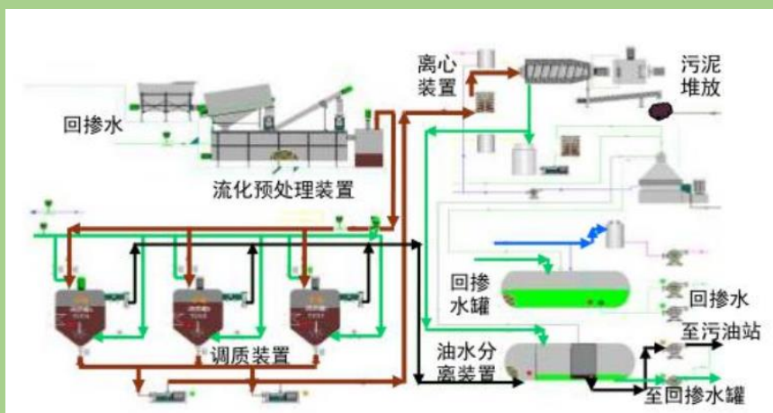
图 3.10-4 朝一联含油污泥处理站工艺流程图
