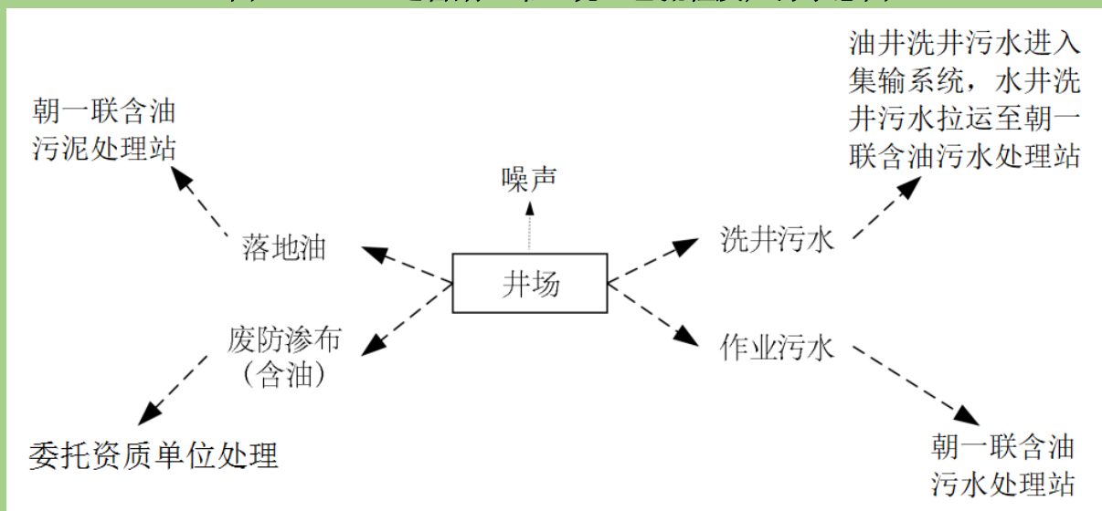
图 3.11-5 运营期正常工况工艺流程及产污示意图
