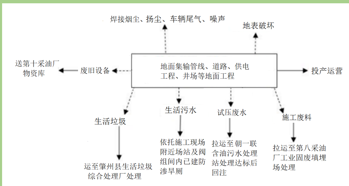
图 3.11-4 本项目地面工程施工期产污环节图
