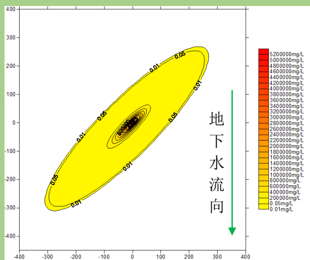
图 5.3-6 油井套管泄漏 5000 天石油类污染扩散平面图（污染源点：0，0）
