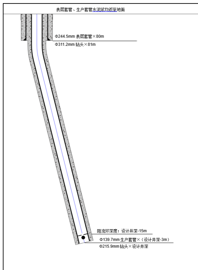
图 3.6-2 定向井井身结构示意图
