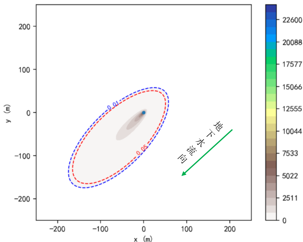
图 5.3-10 油井套管泄漏 5475 天石油类污染扩散平面图（污染源点：0，0）
