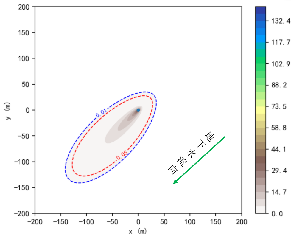
图 5.3-15 注水井套管泄漏 5475 天石油类污染扩散平面图（污染源点：0，0）
