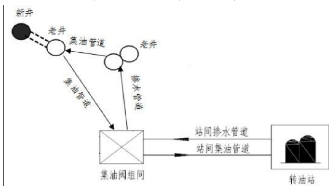
图 3.6-7 单管环状掺水集油工艺示意图
