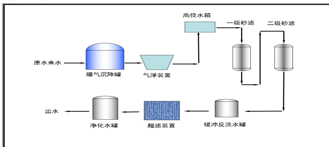
图 3.11-6 朝一联合含油污水处理站工艺流程
