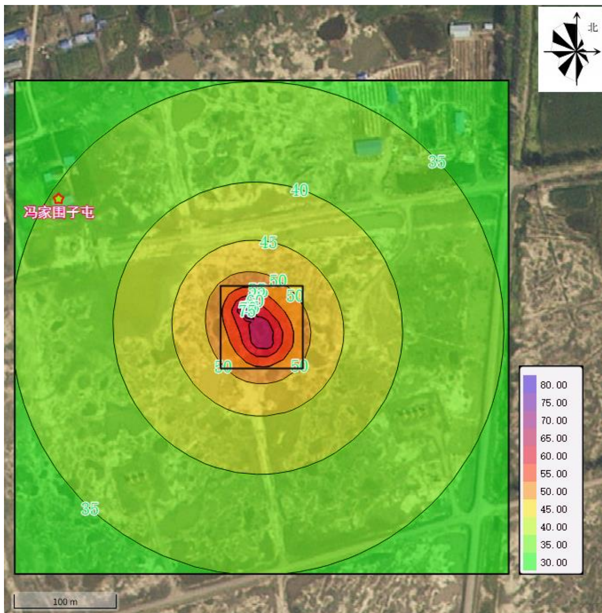
图 5.4-1 朝 119-更 63 钻井工程噪声贡献值预测图
