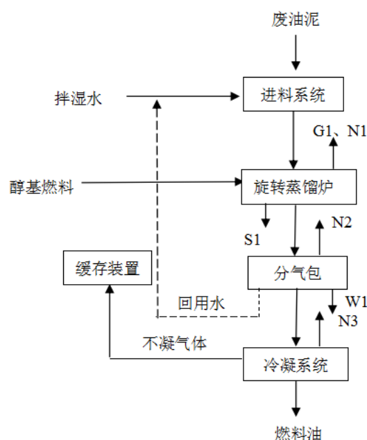
图 3.11-9 大庆博昕晶化科技有限公司工艺流程图
