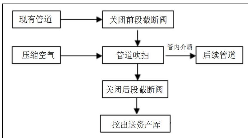
图 3.8-1 原有管道处理流程图
