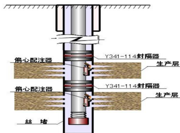
图 5.3-12 全过程一体化分注管柱示意图
