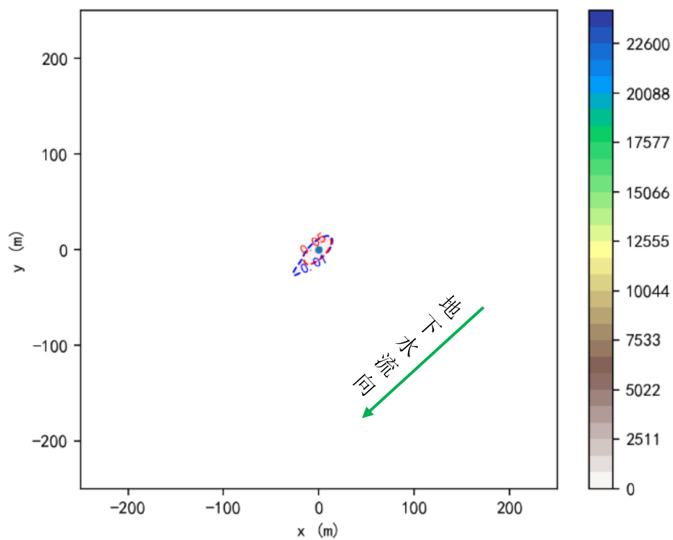
图 5.3-8 油井套管泄漏 100 天石油类污染扩散平面图（污染源点：0，0）
