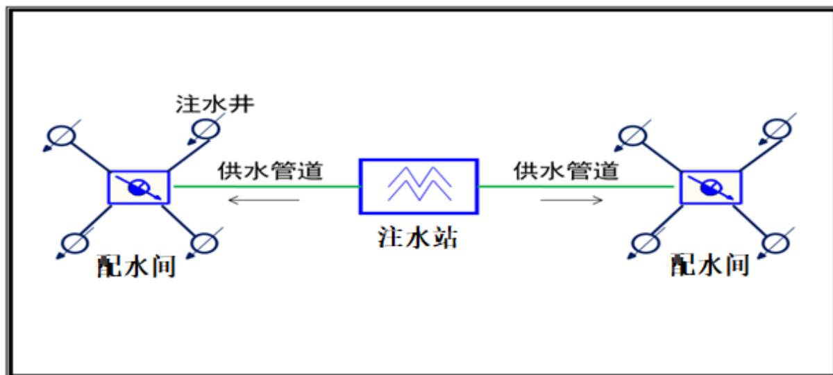
图 3.6-8 本项目注水系统工艺流程图
