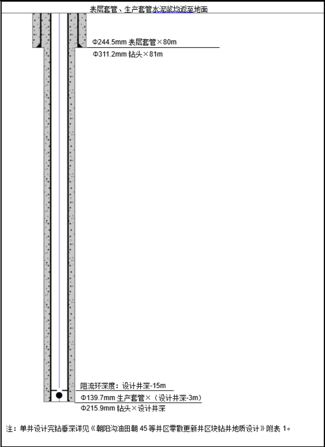
图 3.6-1 直井井身结构示意图
