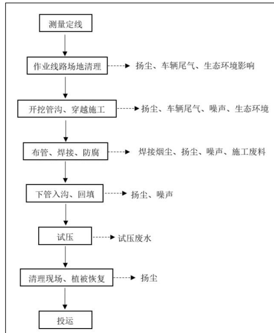
图 3.12-3 管线施工过程示意图
