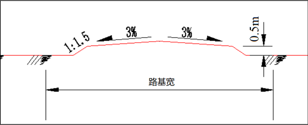
图3.8-7 通井路横断面示意图
