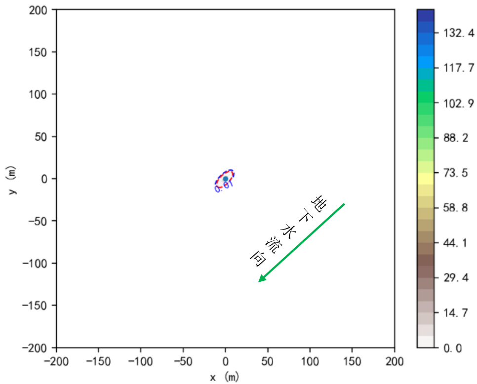
图 5.3-13 注水井套管泄漏 100 天石油类污染扩散平面图（污染源点：0，0）
