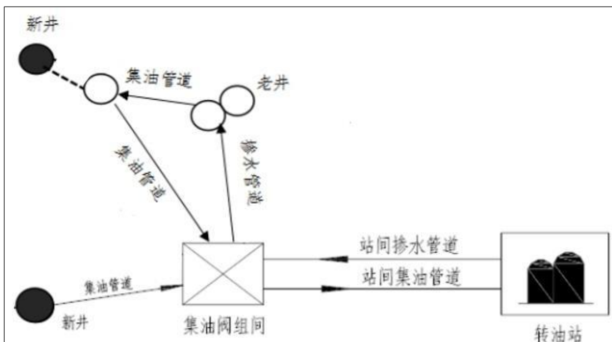
图 3.6-6 电加热集油工艺示意图
