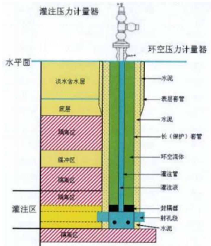
图 5.3-11 注水井井身结构示意图
