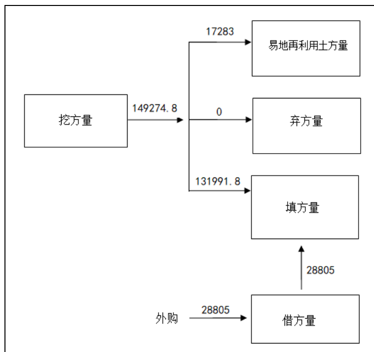
图 3.7-1 土石方平衡图 (单位: \text{m}^3 )
