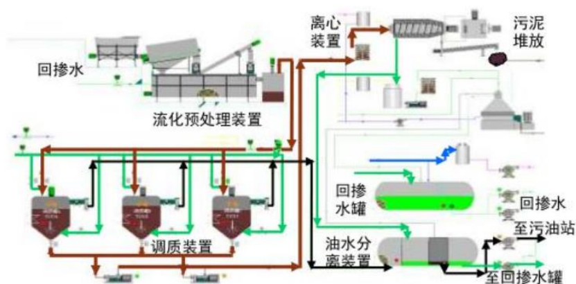
图 3.11-8 朝一联含油污泥处理站工艺流程图
