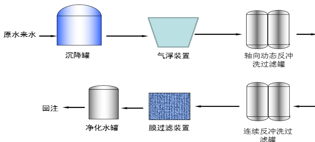
图 3.11-7 朝二联合油污水处理站工艺流程
