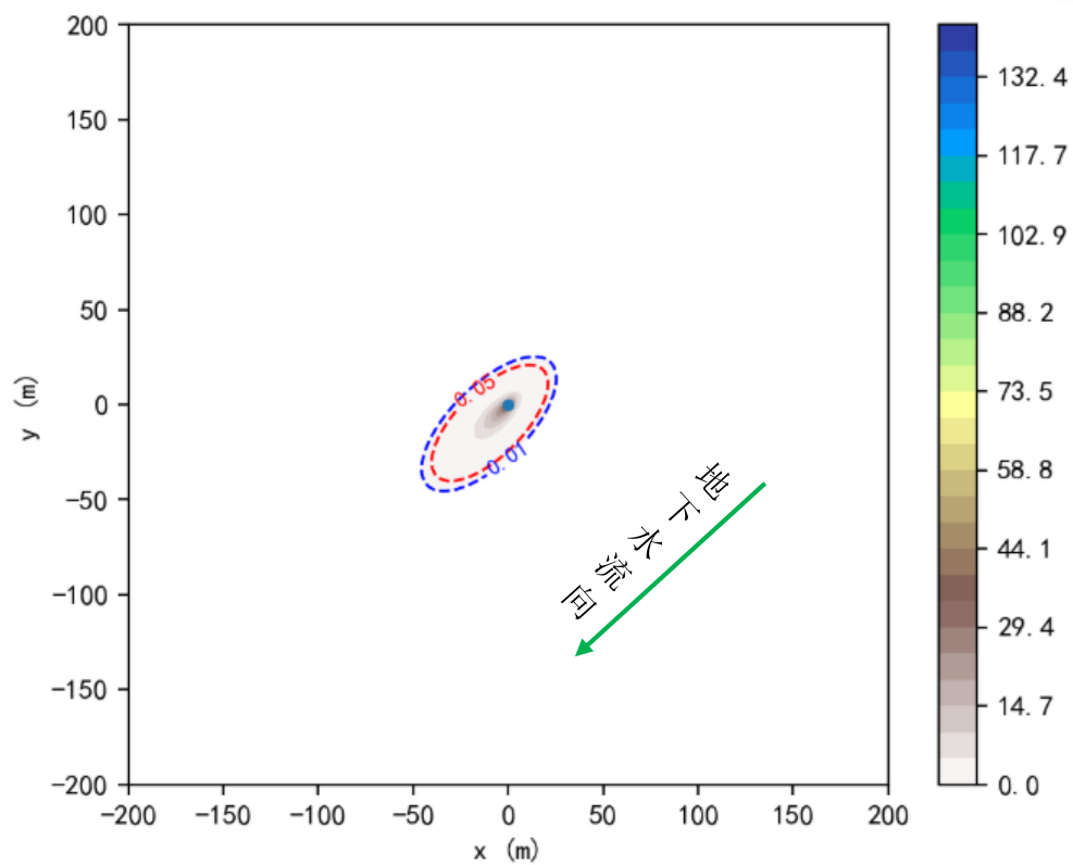
图 5.3-14 注水井套管泄漏 1000 天石油类污染扩散平面图（污染源点：0，0）
