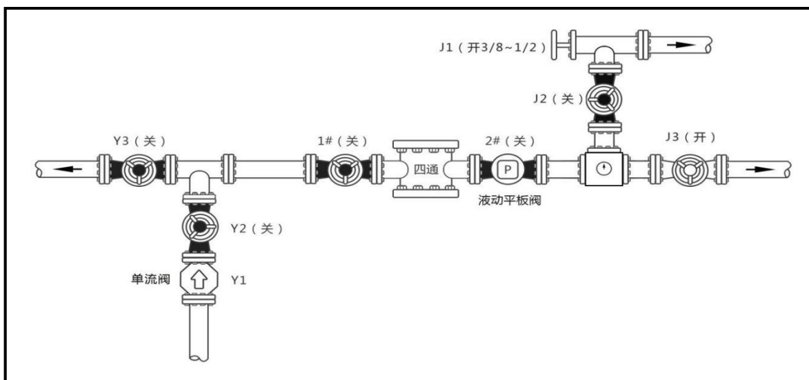
图 3.6-5 二开井口管汇示意图
