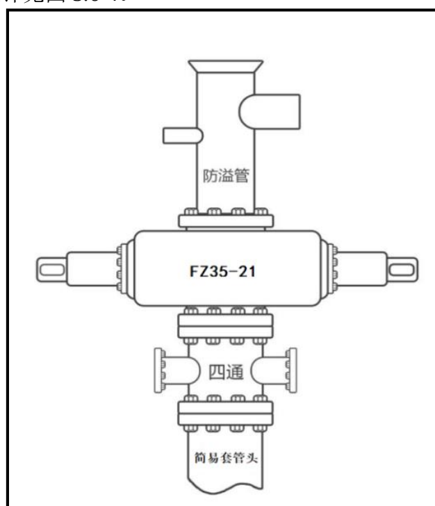
图 3.6-4 二开井口装置示意图
