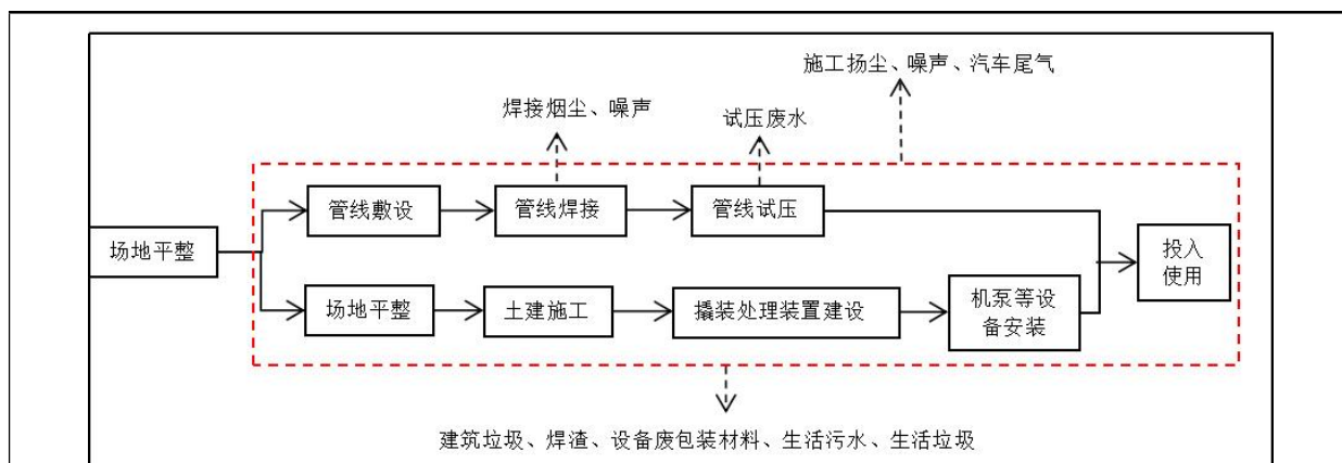
图 2-1 施工期工艺流程及产污节点图
