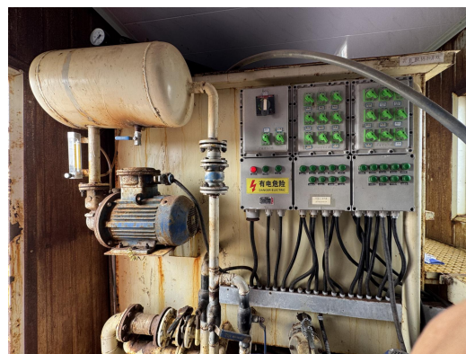
气浮泵
