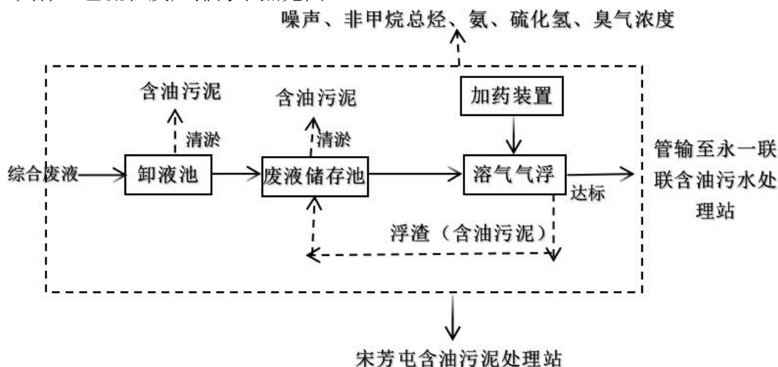
图 2-2 运营期主要工作流程及产污节点图
