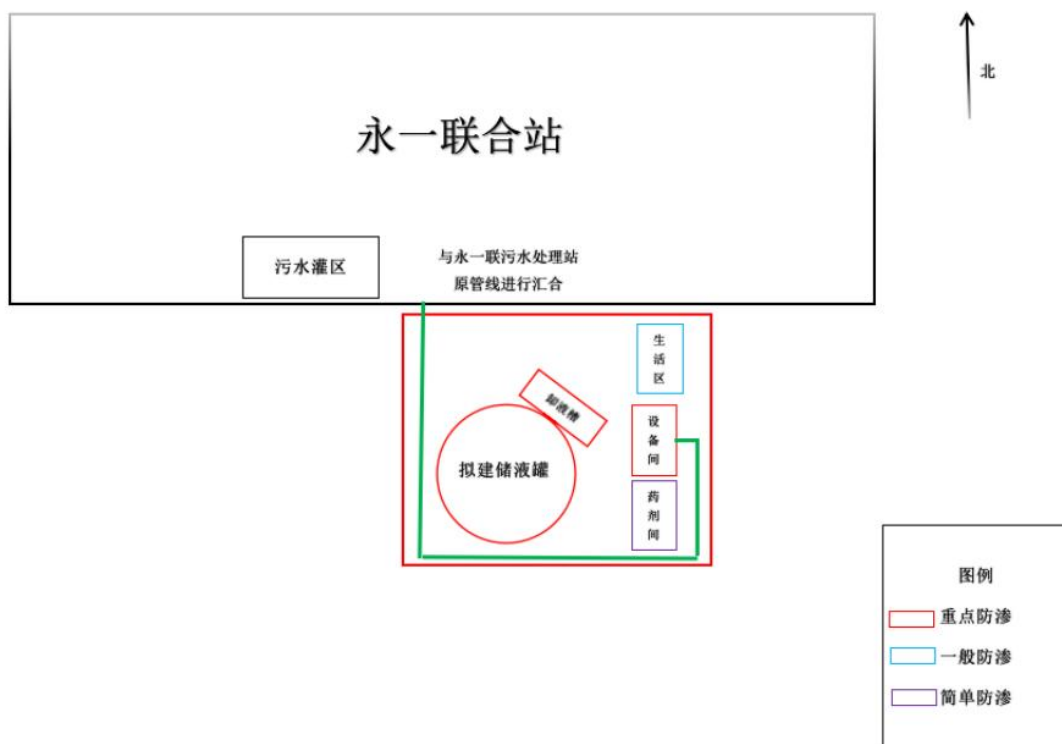
附图 3：平面布置图
