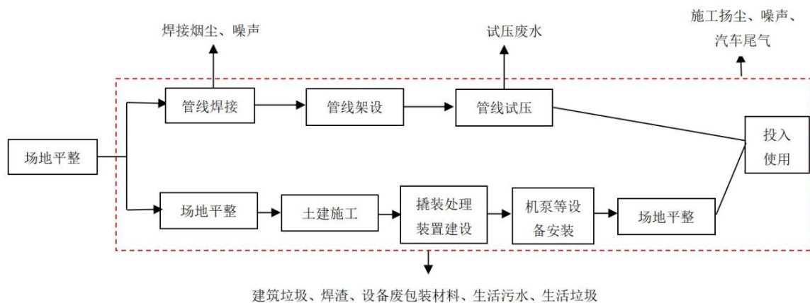
图 2-1 施工期工艺流程及产污节点图
