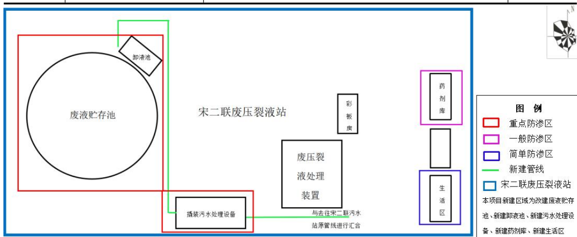
图 3-3 本项目分区防渗图
