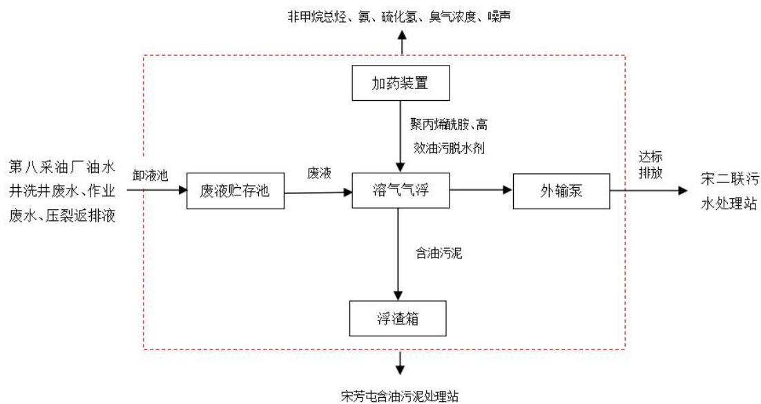
图 2-2 运营期主要工作流程及产污节点图
