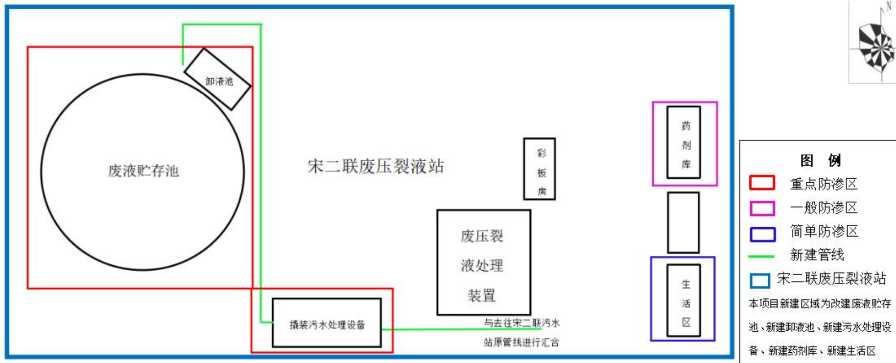
附图 4：分区防渗图
