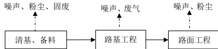
图 3.2-4 道路工程施工流程及排污节点图
