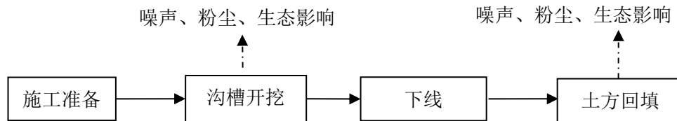
图 3.2-5 农田输配电工程施工流程及排污节点图
