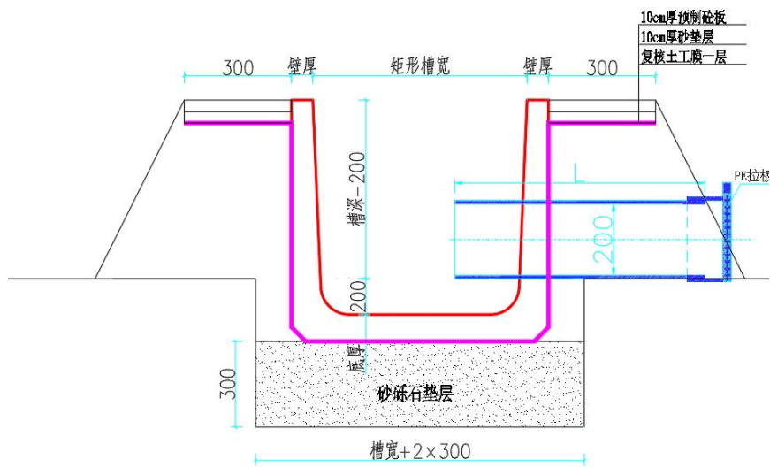
图 3.2-2 砣矩形槽护砌示意图
