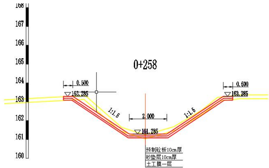
图 3.2-1 砣板护坡方案示意图
