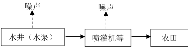
图 3-2-10 灌溉井工艺流程及排污节点图
