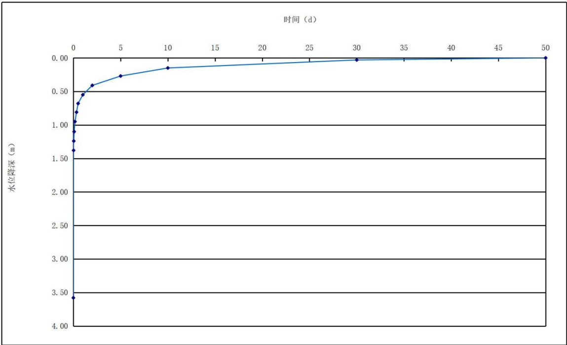
图 5.2-1 地下水中心水位降深恢复动态
