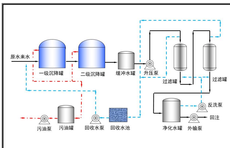
图 3.6-1 卫一联合含油污水深度处理站工艺流程图
