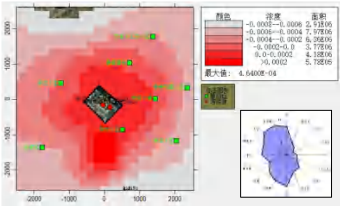
图 5.1-7 SO 2 年平均质量浓度分布图
