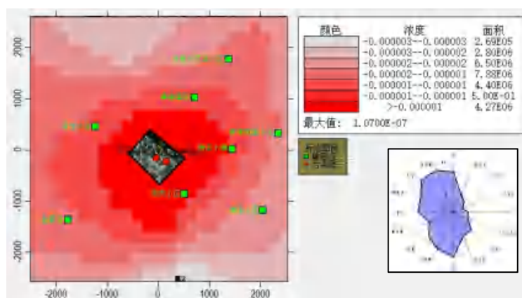
图 5.1-9 \text{NO}_2 年平均质量浓度分布图
