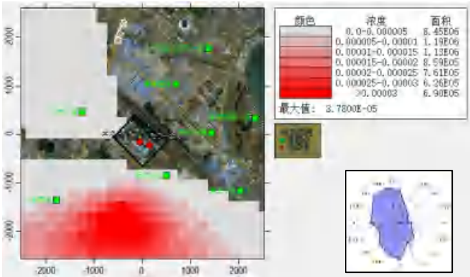
图 5.1-6 SO 2 日平均质量浓度分布图
