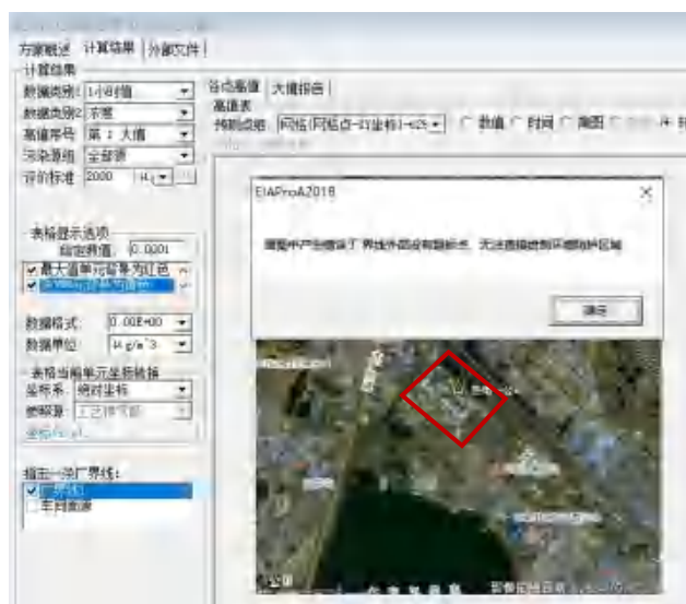
图 5.1-21 本项目 NMHC 防护距离计算结果图 ( \mu\text{g}/\text{m}^3 )
