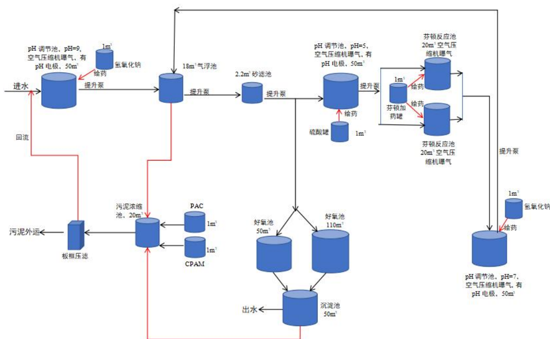
图3.1-1 污水站工艺流程图
