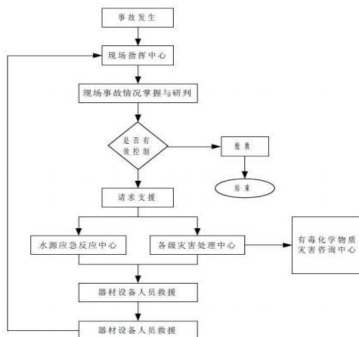
图5.3-1 事故应急流程
