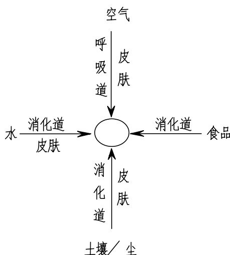
图5.4-1 人体经各环境介质暴露污染物的途径
